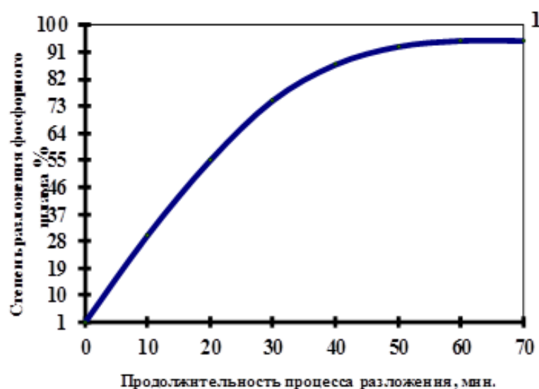
Рис. 2. Зависимость степени разложения фосфорного шлама от продолжительности проведения процесса при 60°C
