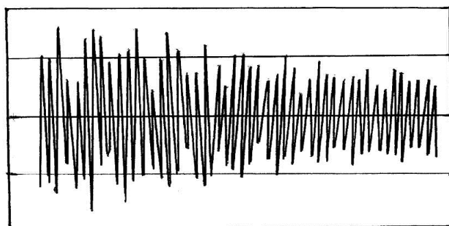
2-сурет. 30 ХС болат үлгісінің соққыш-шар екпінінен дыбыс импульсінің азаю осциллограммасы келтірілген
