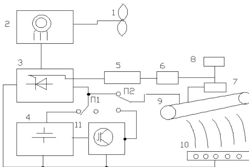
Рис. 1. Станция катодной защиты: 1 – ветродвигатель; 2 – генератор; 3 - силовая часть управляемого выпрямителя; 4 – буферные аккумуляторы; 5 – СИФУ; 6 – регулятор; 7 – контрольно-измерительный пункт; 8 - устройство задания; 9 – газовая труба; 10 – анодный заземлитель; 11 – широтно-импульсный регулятор; П1, П2 переключатели.
