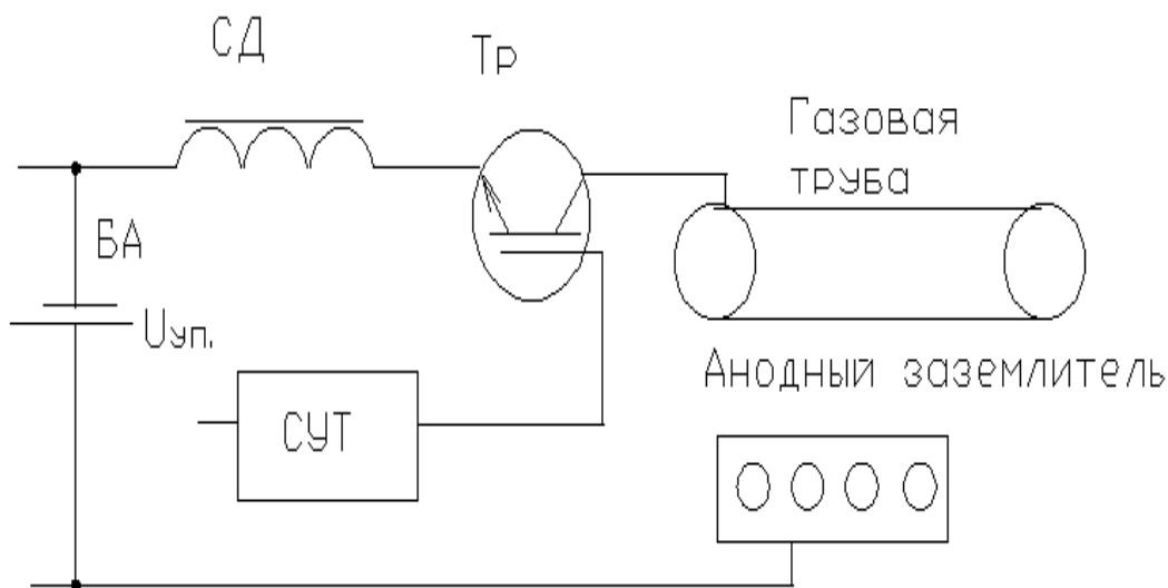
Рис. 5. Схема силовой части импульсного регулятора постоянного напряжения
