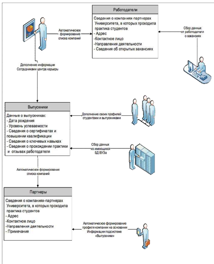
Рис. 3. Схема потоков данных
