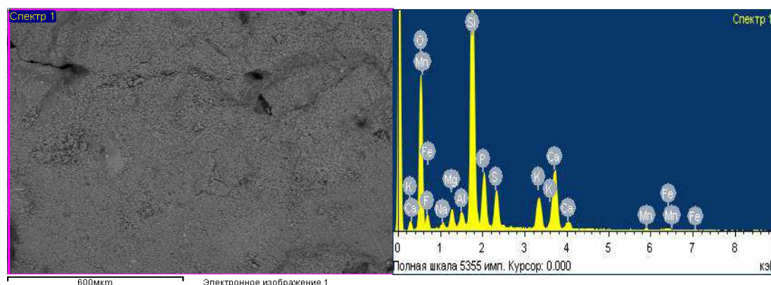
Рис. 4. Минерологический состав и микроструктура образца комплексного полимерсодержащего удобрения суперфосфата
