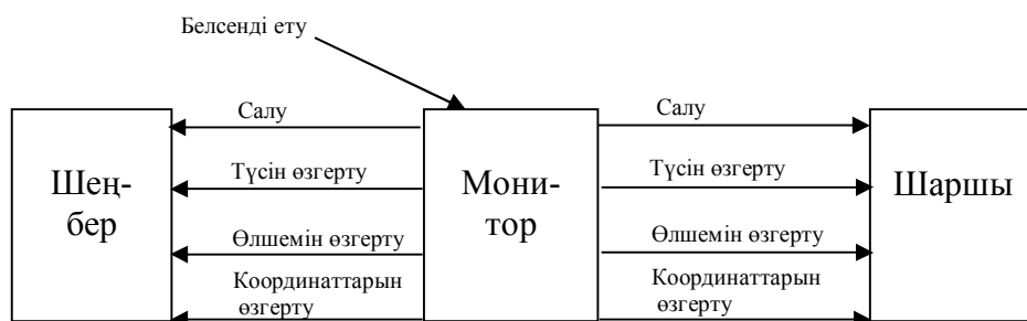
4-сурет. Графикалық редактор объектілерінің диаграммасы
