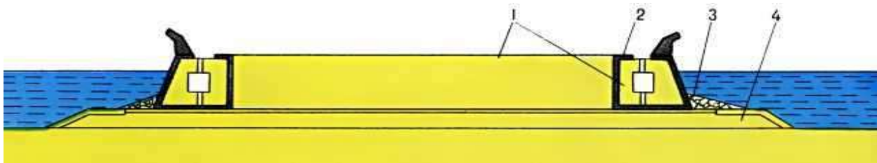
Рис. 3. Остров с железобетонным кессонным ограждением: 1 - песок; 2 - железобетонный кессон; 3 -каменная наброска; 4 - гравийно-песчаная смесь.
