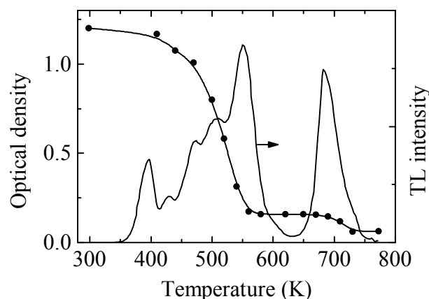
Рис. 4. Зависимость радиационно-индуцированного оптического поглощения от температуры промежуточных нагревов для полосы при 2.21 эВ ( \bullet ) и кривая ТСЛ (правая шкала) для облученного при комнатной температуре ионами \text{Xe}^{132} с флюенсом 1 \times 10^{14} ион/см 2 кристалла \text{CaF}_2 . Оптическое поглощение измерено при комнатной температуре.
