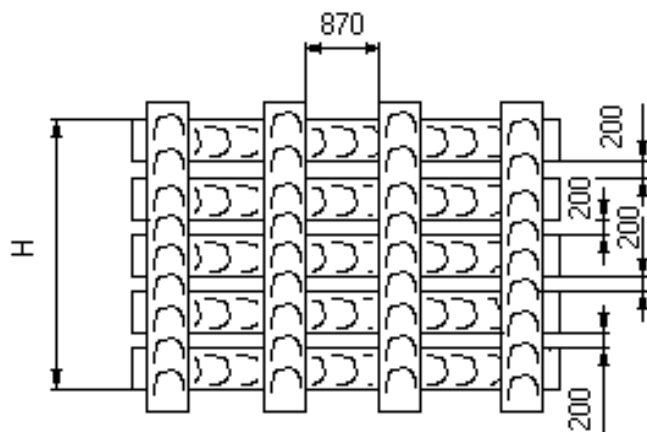
Рис.1.3. Деревянный щит ограждения
