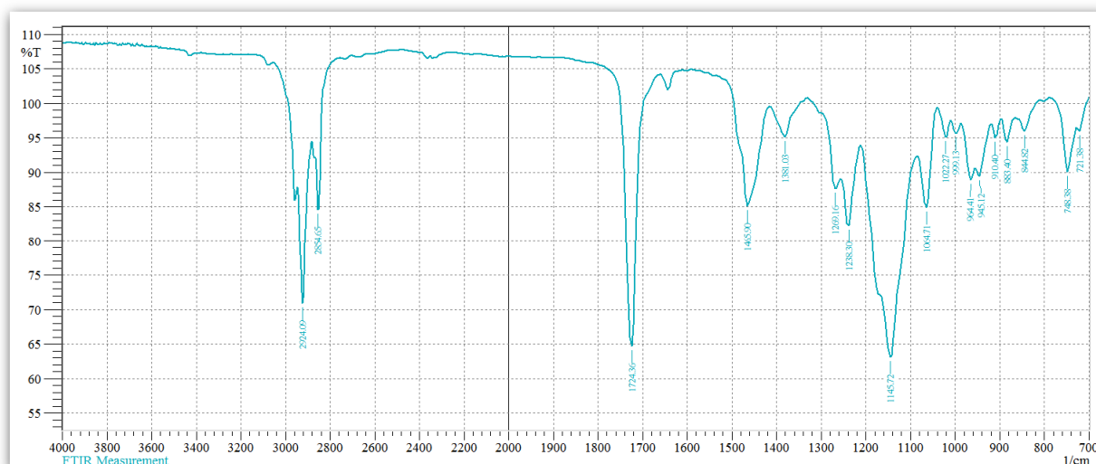
Рис. 6. ИК- спектр тройного сополимера
