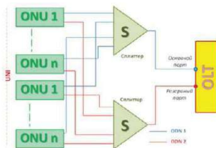
Рис. 2.4. Схема резервирования. Тип С
