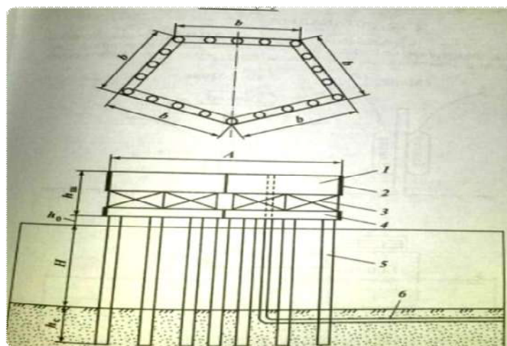
Рис.6. Насыпной остров с двухпалубной конструкцией.
