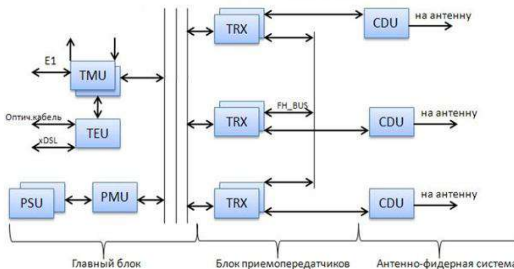
Рис. 2. Структурная схема базовой станции
