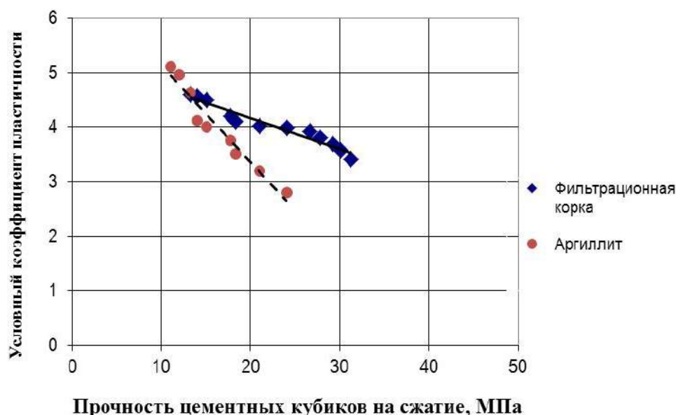
Рис. 6. Условный коэффициент пластичности при испытании образцов тампонажного камня на приборе УМП – 3
