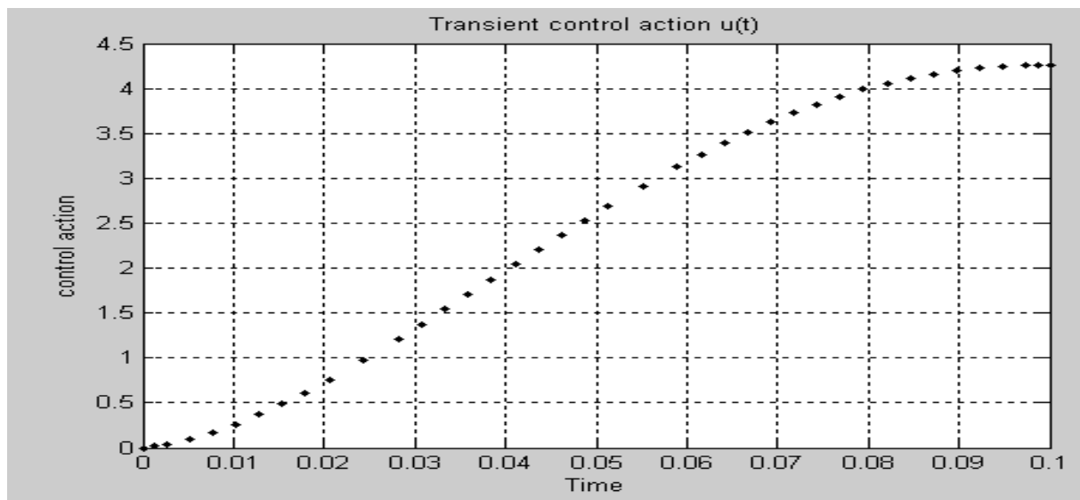
Рис. 2. Кривая переходного процесса оптимального управления замкнутой системы ПЧ – АД
