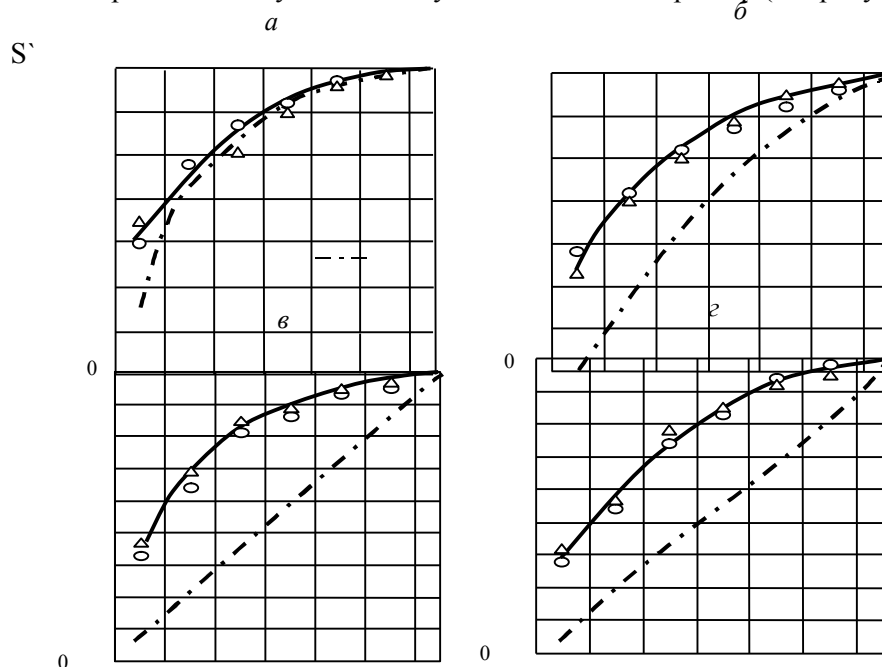
Рис. 2. Динамика параметров нерабочего борта Житикаринского карьере
