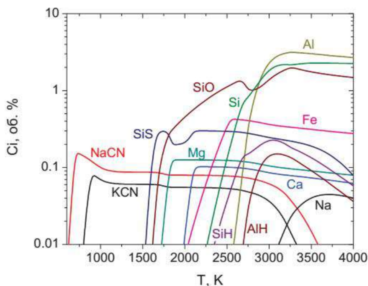
Рис. 3. Температурная зависимость концентраций минеральных компонентов в газовой фазе при комплексной переработке угля
