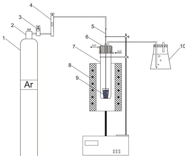
1-сурет. Шлактарды кедейлендірудің тәжірибелік құрылғысының сұлбасы 1 – аргоны бар баллон; 2 – газды вентиль; 3 – газды редуктор; 4 – ротаметр; 5 – үрлеу түтікшесі; 6 – сумен суытылатын тығын; 7 – кварцты реактор; 8 – құбырлы қыздыру пеші; 9 – балқымасы бар тигель; 10 – Дрексельдысы.
