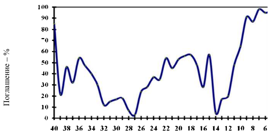
Рис. 5. ИК-спектр полимерсодержащих комплексных удобрений суперфосфата
