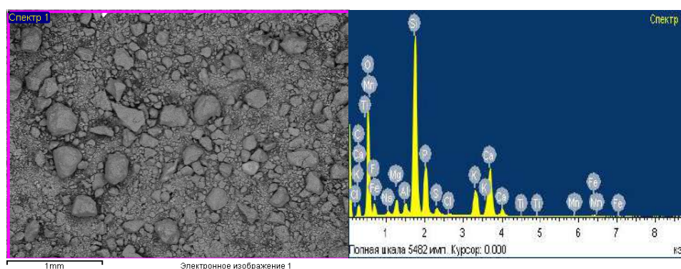
Рис. 1. Минералогический состав и микроструктура фосфорного шлама
