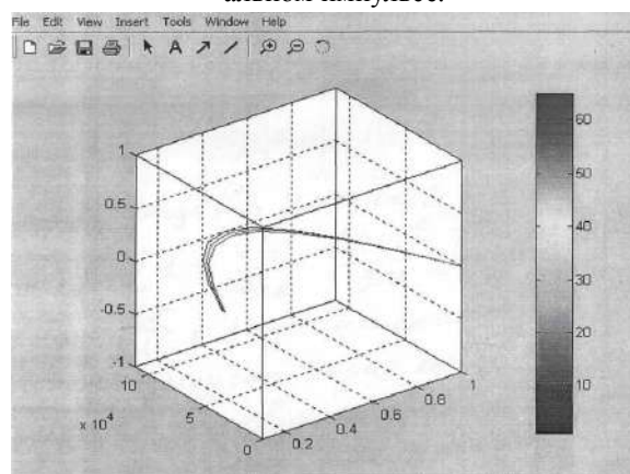
График 4. Характер движения деформации материала площади контакта в плоскости X-Z при радиальном импульсе.
