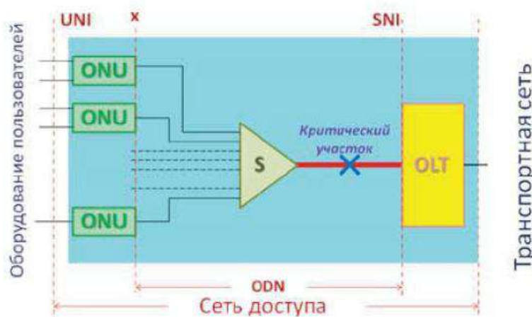
Рис. 2. Надежность PON. Критический участок
