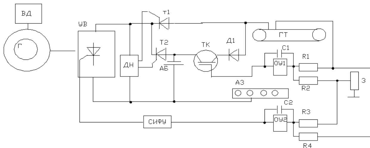
Рис. 2. Схема катодной защиты с питанием от двух источников:
