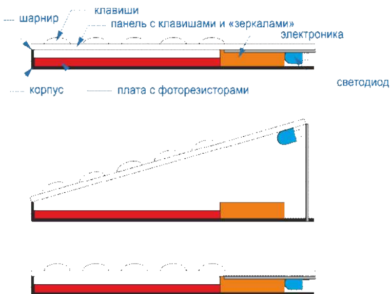
Рис. 1. Схематическое изображение клавиатуры в рабочем и не рабочем состоянии
