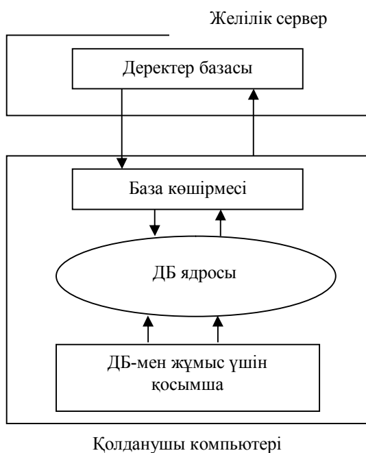
1-сурет. «Файл-сервер» архитектурасы
