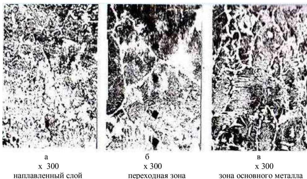
Рис. 1. Микроструктура наплавленного металла (образец «1», коренная шейка, 15 ГЮСТЦА +порошок)
