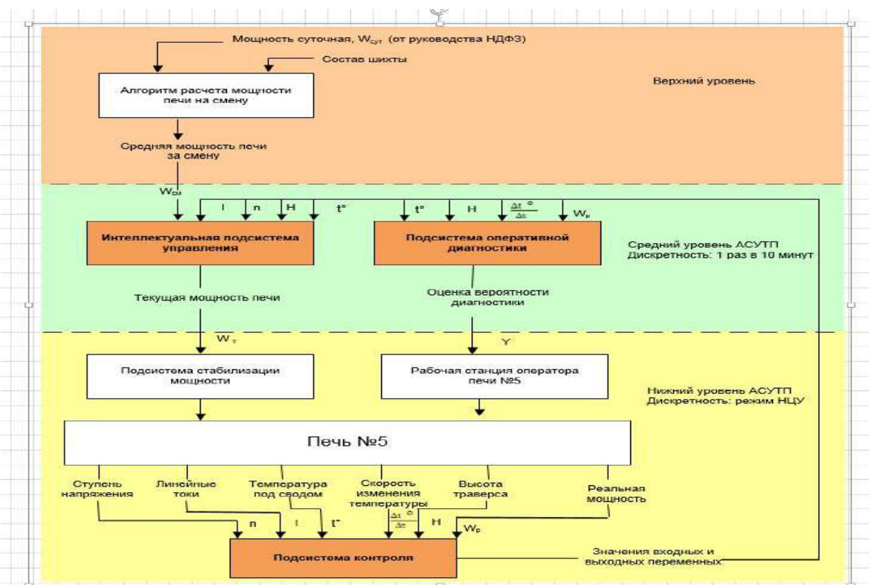
Рис. 1. Трёхуровневая иерархическая структура системы оптимального управления процессом производства желтого фосфора
