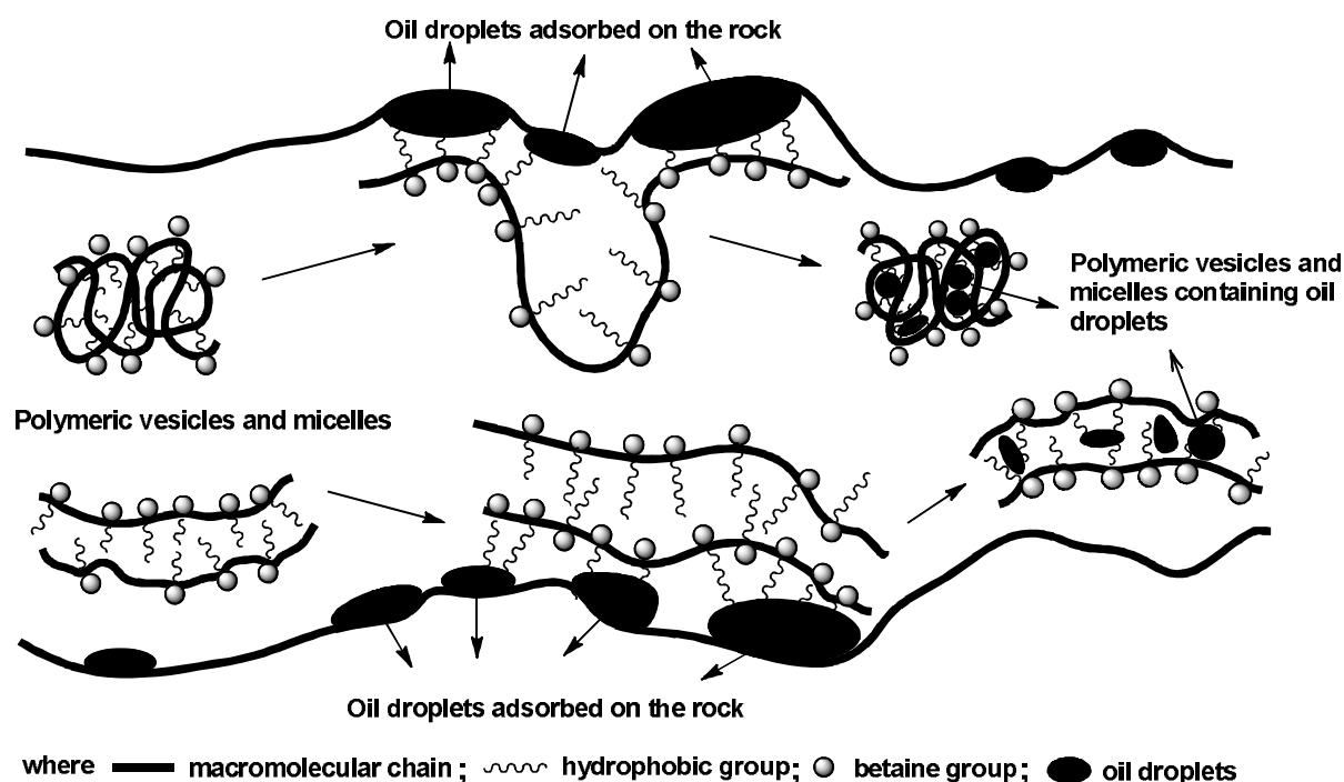
Рис. 2. Механизм процесса вытеснения нефти при применении АСП заводнения
