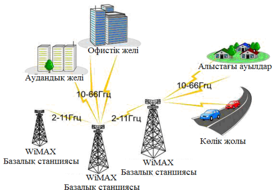
4-сурет. Станция мен антеналар арасындағы байланыс жиіліктері
