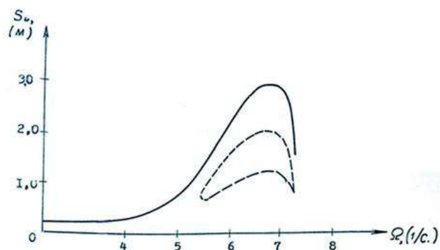
Рис. 4. Амплитудно-частотная характеристика колебаний нити на частоте суммарного тона при \gamma=2
