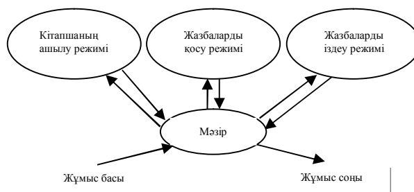
5-сурет. Қолданушы интерфейсі жағдайының диаграммасы.
