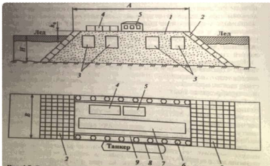
Рис.5. Островное нефтегазовое сооружение массивной формы.
