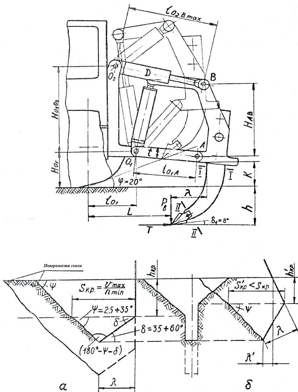
Рис. 1. Схема синтеза четырехзвенного рыхлителя с минимальными реакциями в звеньях
