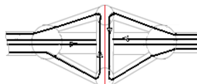
б. Развязка типа двойная подкова
