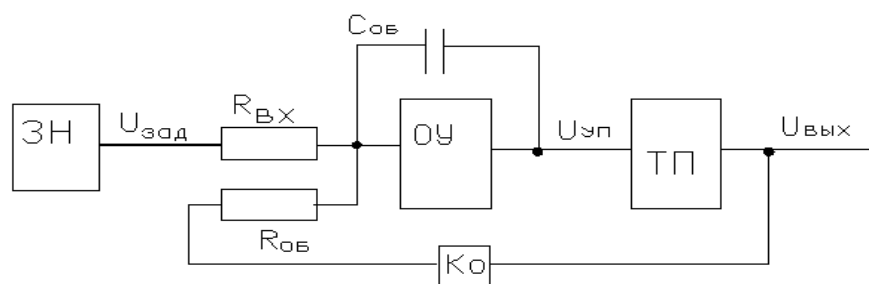
Рис. 3. Функциональная схема системы стабилизации отрицательного напряжения на газовой трубе
