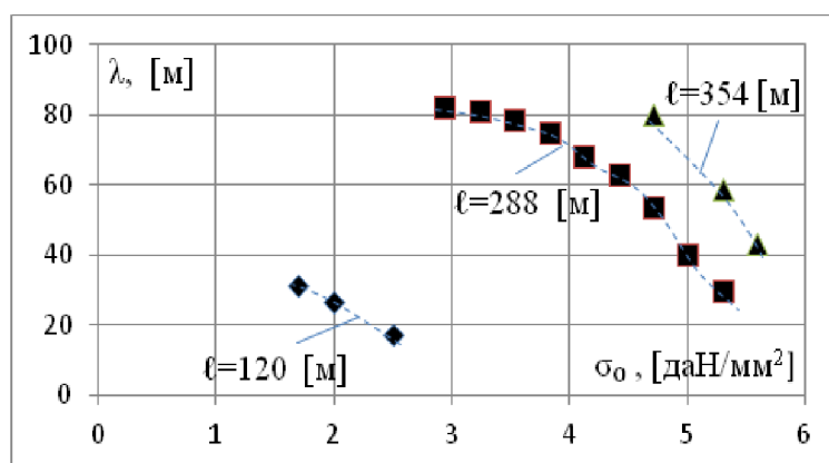
Рис. 6. Экспериментальная зависимость \lambda (м) от \sigma_0 (даН/мм²)
