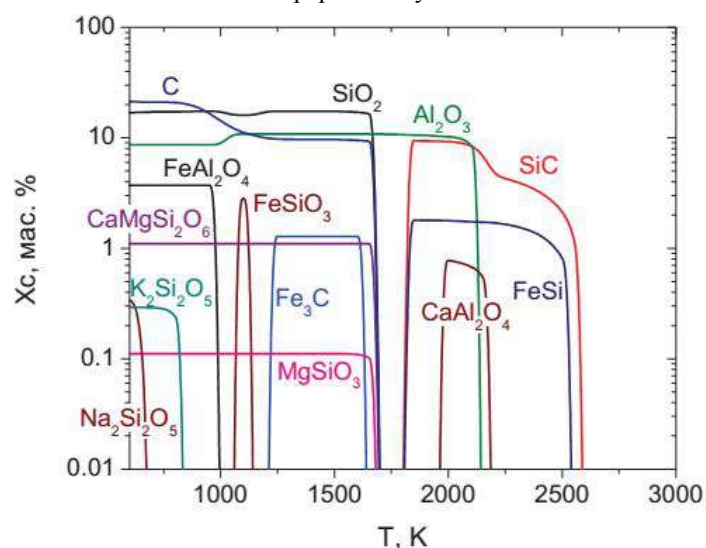
Рис. 4. Температурная зависимость концентраций компонентов конденсированной фазы при комплексной переработке угля
