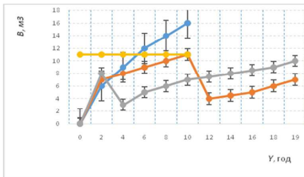
Рис. 4. График зависимости объемов вскрыши и длины фронта горных работ от периода разработки, построенный для Житикаринского карьера
