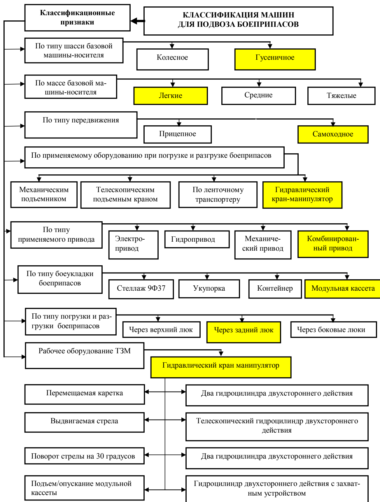
Рис. 6. Классификация транспортно-заряжающих машин
