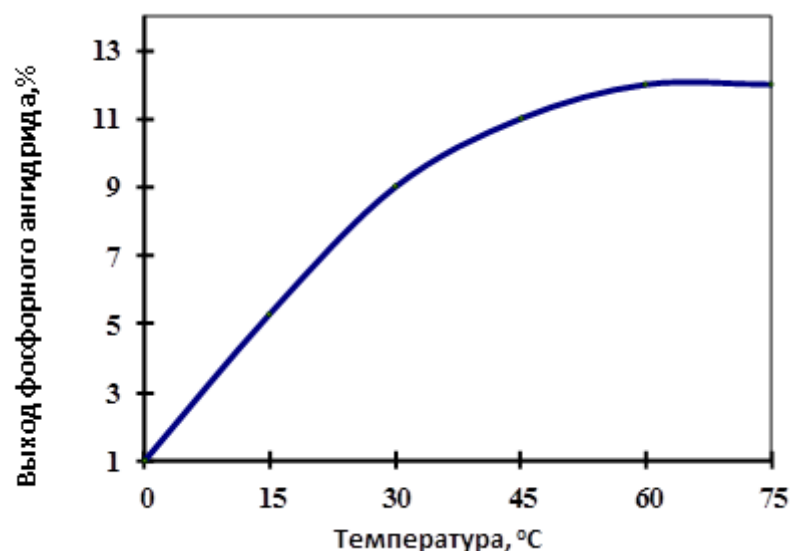
Рис. 3. Зависимость выхода фосфорного ангидрида от температуры при разложении фосфорного шлама
