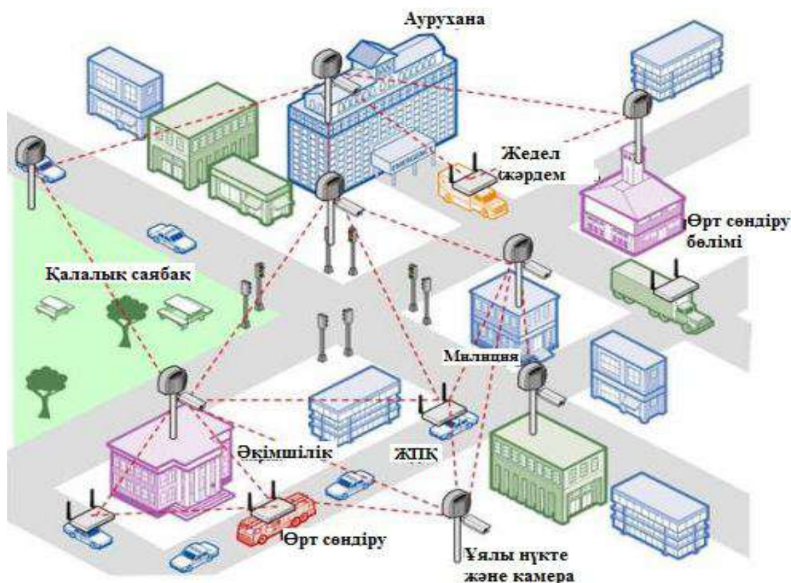
2-сурет. MESH -желісінің қаладағы кездейсоқ жағдайларда қолданылуы
