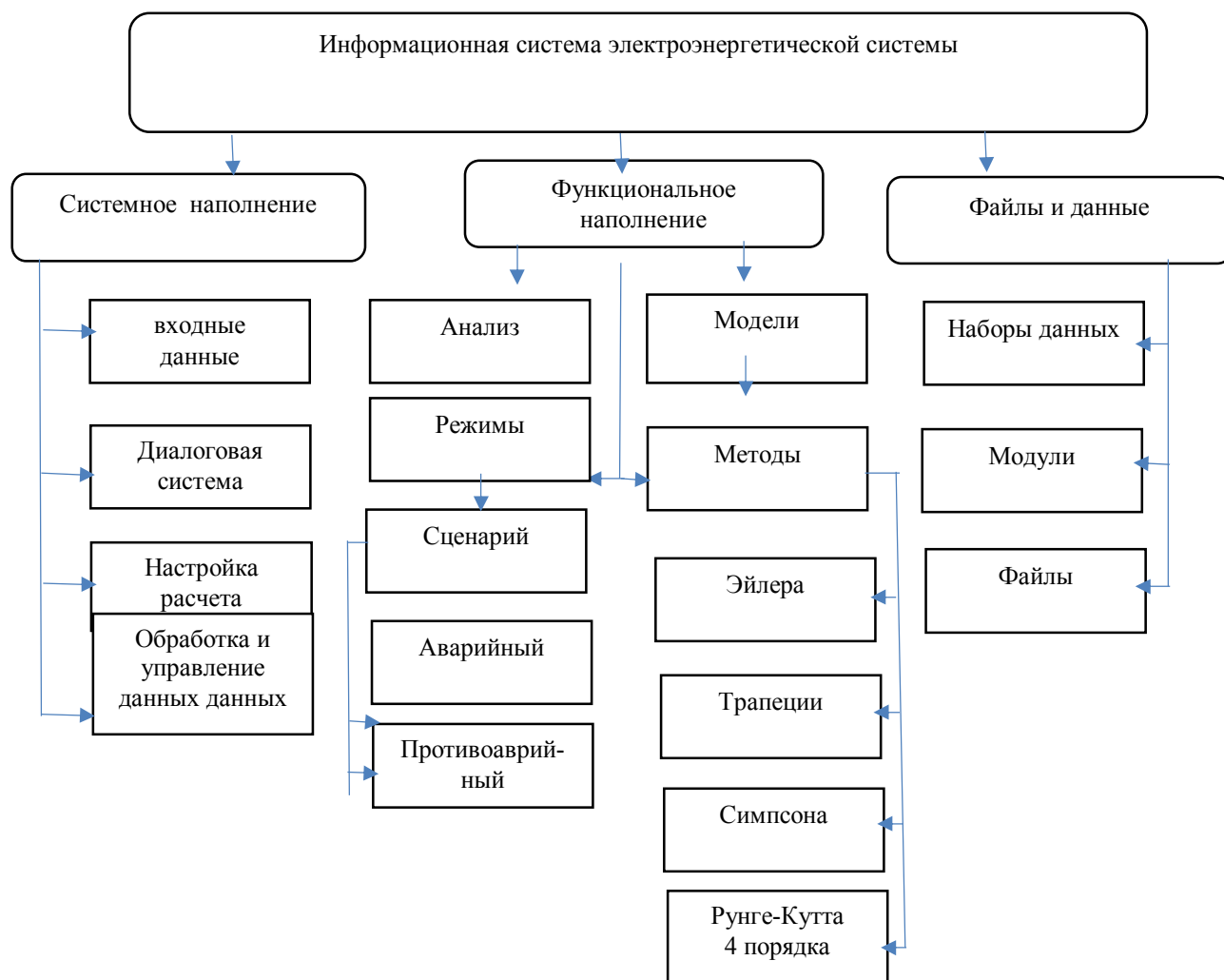
Рис. 1. Общая структура информационной системы.
