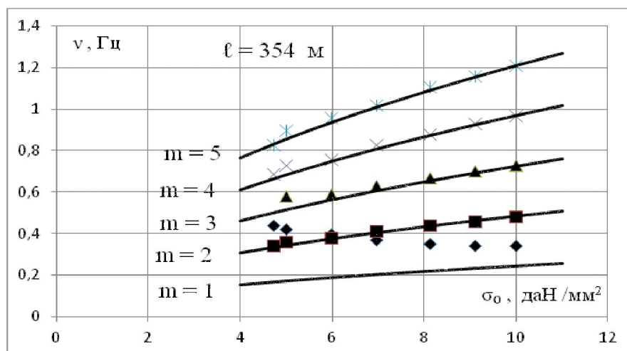
Рис. 3. Зависимость частоты от начального напряжения и числа полуволн.
