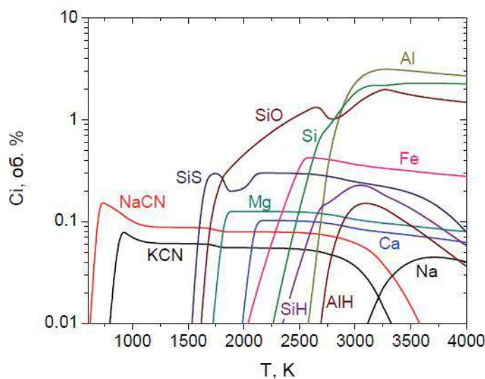
Рис. 2. Температурная зависимость концентраций минеральных компонентов в газовой фазе при плазменной газификации ККУ (с учетом кислорода ММУ)
