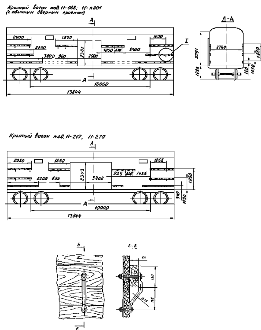
Рис. 1.2. Расположение деталей несъемного оборудования внутри кузова крытого вагона
