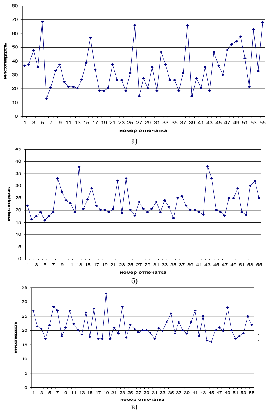
Рис. 2. Значения микротвердости исследуемых образцов: а) образец А; б) образец Б; в) образец В
