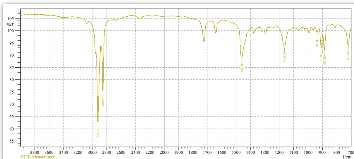
Рис. 5. ИК-спектр сополимера бутилметакрилата и винилацетата
