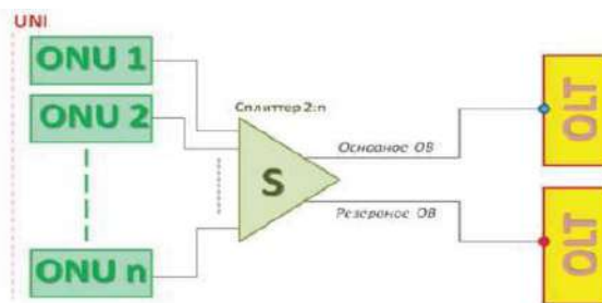
Рис. 2.3. Схема резервирования. Тип В с двойным ОLT
