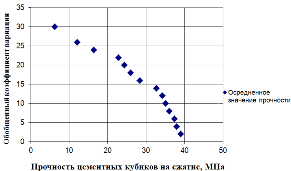
Рис. 7. Значения обобщенного коэффициент вариации при испытании образцов тампонажного камня на одноосное сжатие
