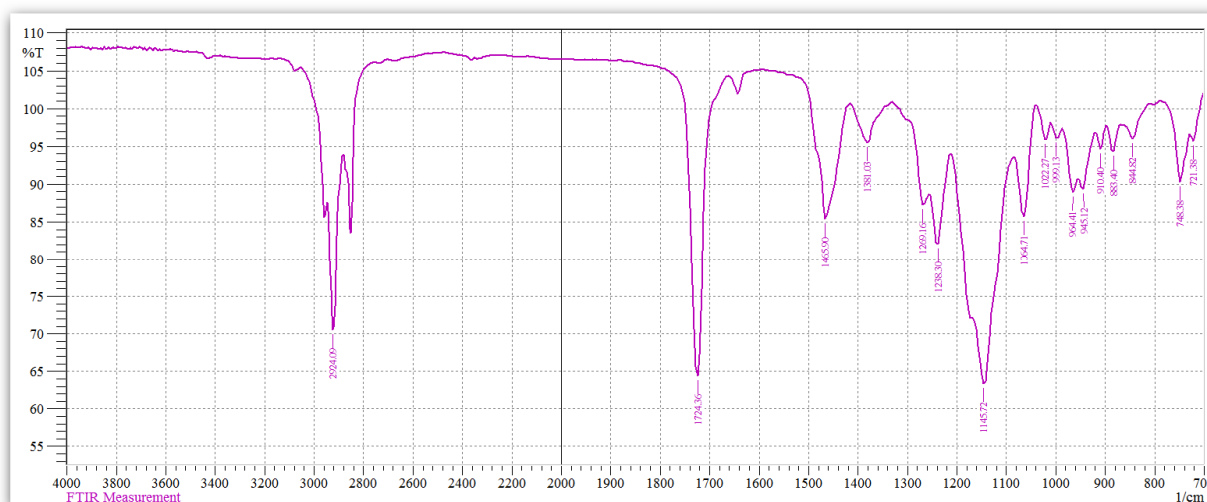
Рис. 4. ИК-спектр сополимера бутилметакрилата и \alpha -олефина
