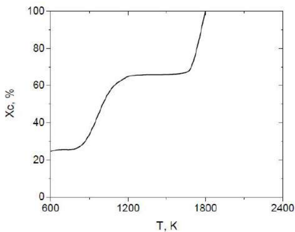
Рис. 5. Температурная зависимость степени газификации угля на процесс плазменной газификации (с учетом кислорода ММУ)
