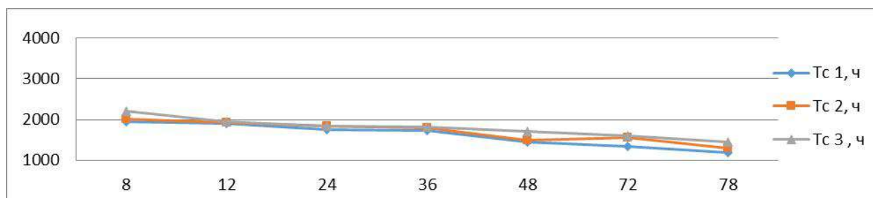
Рис. 3. Зависимость средней наработки на отказ от времени восстановления
