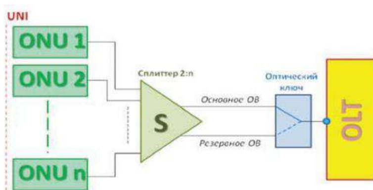
Рис. 2.1. Схема резервирования. ТипА
