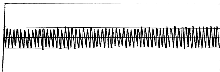
3-сурет Хром-молибден болатының БА - 4 соққыш-шардың екпіні әсерінен дыбыс импульсінің азаю осцилограммасы көрсетілген
