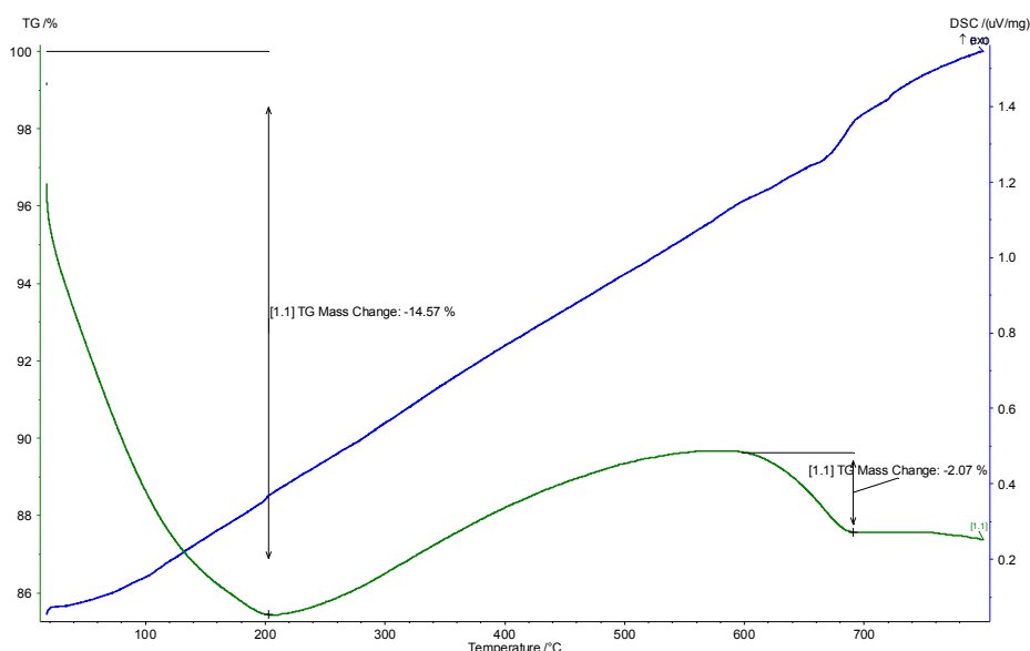
Рис. 3. Дериватограмма диспергированного в течение 10 минут фосфорита Каратау
