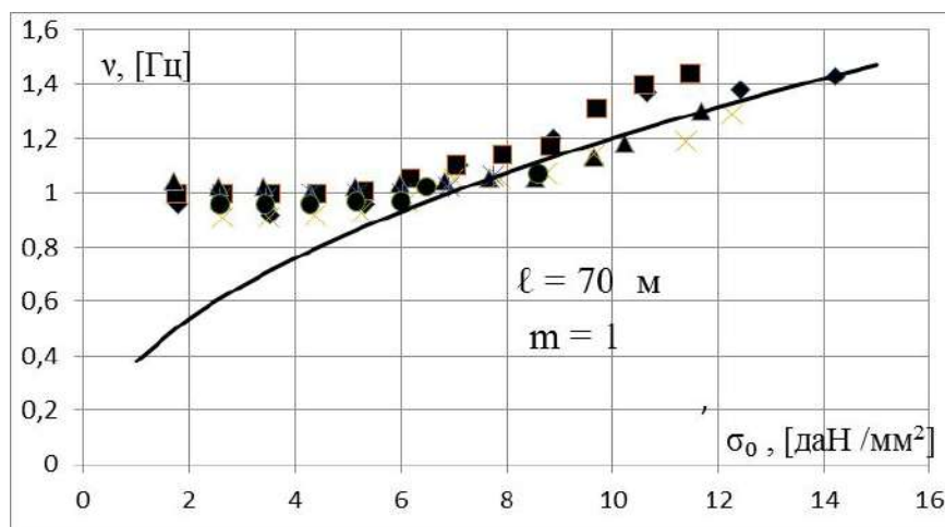
Рис. 4. Зависимость частоты от напряжения: Экспериментальные точки: ◇ - AC-50/8; □ - AC-70/11; △ - AC-95/16; × - AC-120; * - AC-150; ○ - AC-185; Сплошная линия – теоретическая частота
