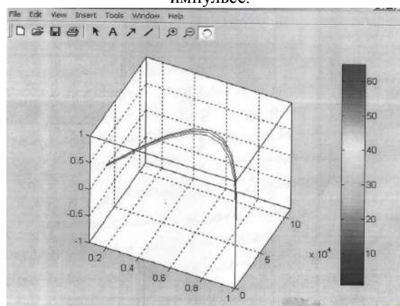
График 3. Характер движения деформации материала площади контакта в плоскости X-Z при линейном импульсе.
