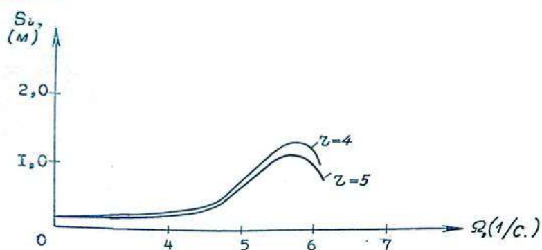
Рис. 6. Амплитудно-частотные характеристики колебаний нити на частоте суммарного тона при \gamma=4 и \gamma=5
