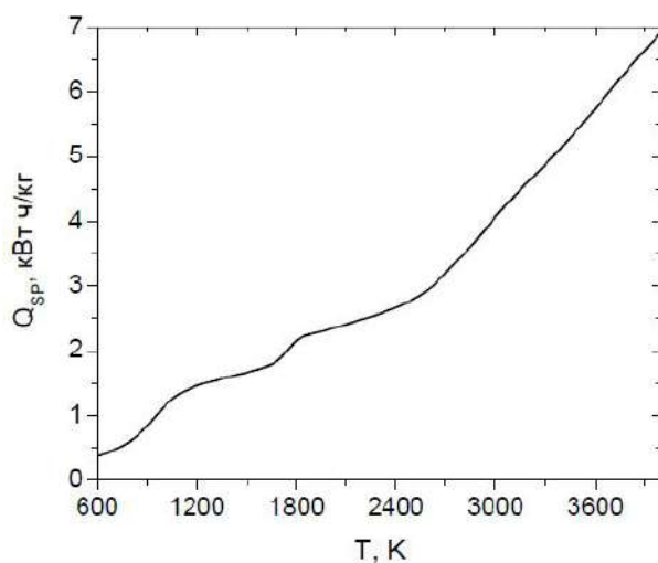
Рис. 4. Температурная зависимость удельных энергозатрат на процесс плазменно-паровой газификации (с учетом кислорода ММУ)
