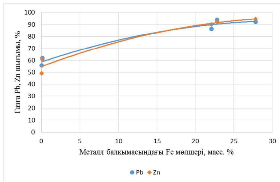
6-сурет. Қорғасынмен мырыштың газға шығарылуының металл балқымасындағы темірдің мөлшеріне тәуелділігі
