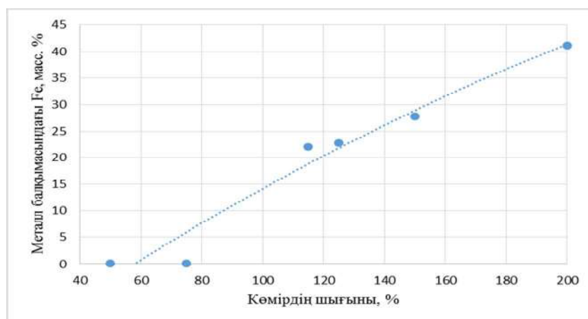
3-сурет. Металл қорытпасына темірдің өтуінің тотықсыздандырғыш шығынынан тәуелділігі
