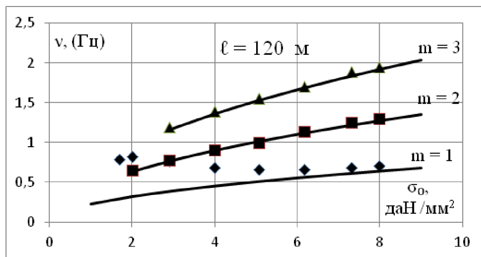
Рис. 1. Зависимость частоты от начального напряжения и числа полувольт Экспериментальные точки:
