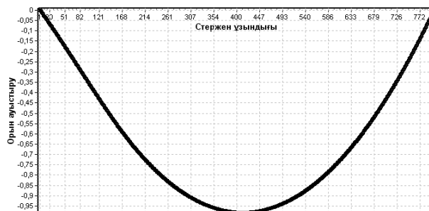
1.3-сурет. Сырық ұзындығы бойынша түйін нүктелердің жылжу заңдылығы
