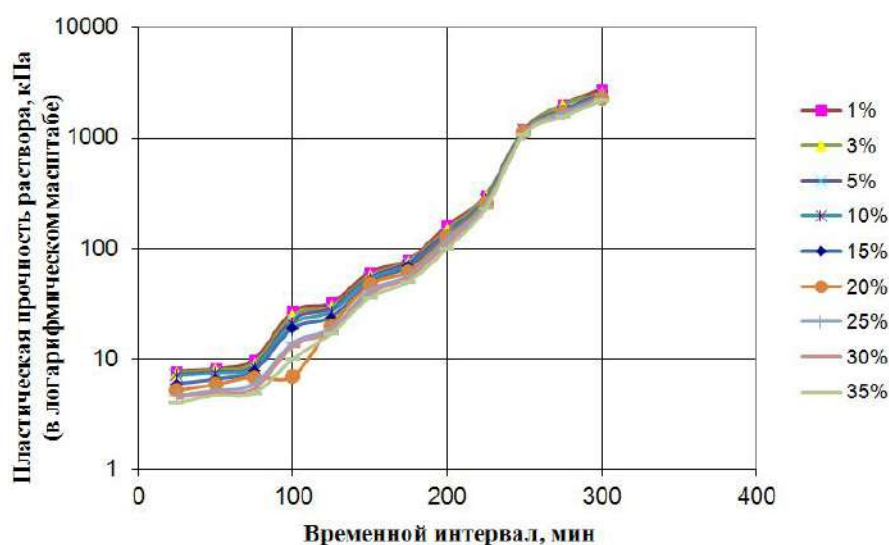
Рис. 1. Изменение пластической прочности тампонажного раствора при введении в него каолиновой глины
