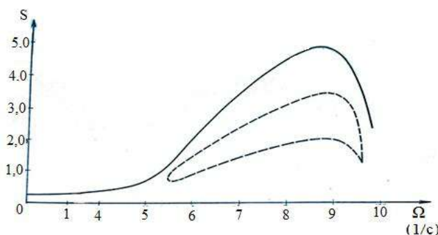
Рис. 3. Амплитудно-частотная характеристика колебаний нити на частоте суммарного тона при r=1
