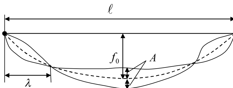
Рис. 5. Форма однополуволнового колебания провода в анкерном пролете при слабых натяжениях
