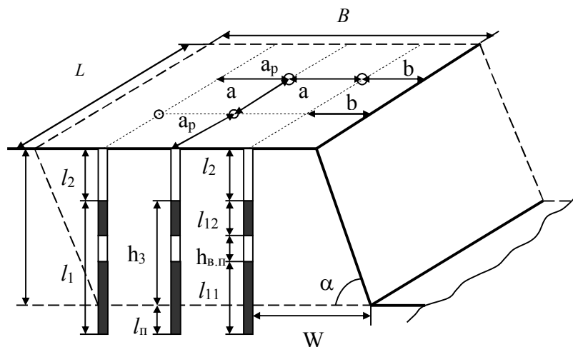
1-сурет. ЖЗ массивте орналасу параметрлері
