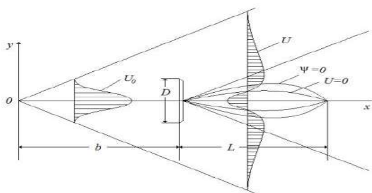
Рис. 1. Схема картины течения, образованного при наложении турбулентной струи-стока на струи-источник
