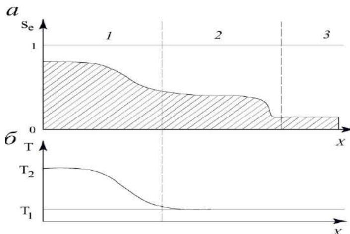
1-сурет. Мұнайдың жеңіл фазаларының булануының болмау жағдайында ыстық сумен мұнайдың бір өлшемді ығыстырылуы кезіндегі температура (б) және сумен қанығу (а) профильдері [4].
