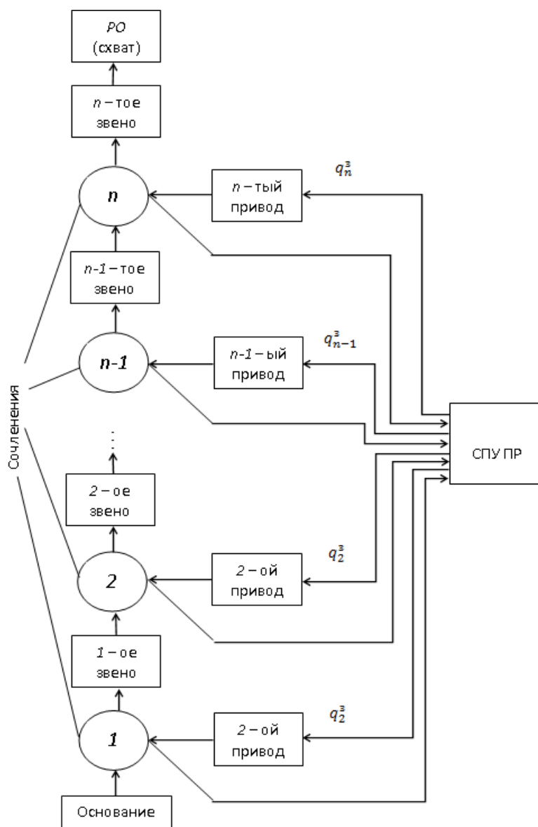
Рисунок 1. – Структурная схема промышленного робота
