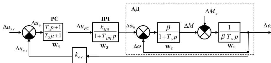
Рис. 1. Структурная схема системы ПЧ-АД
