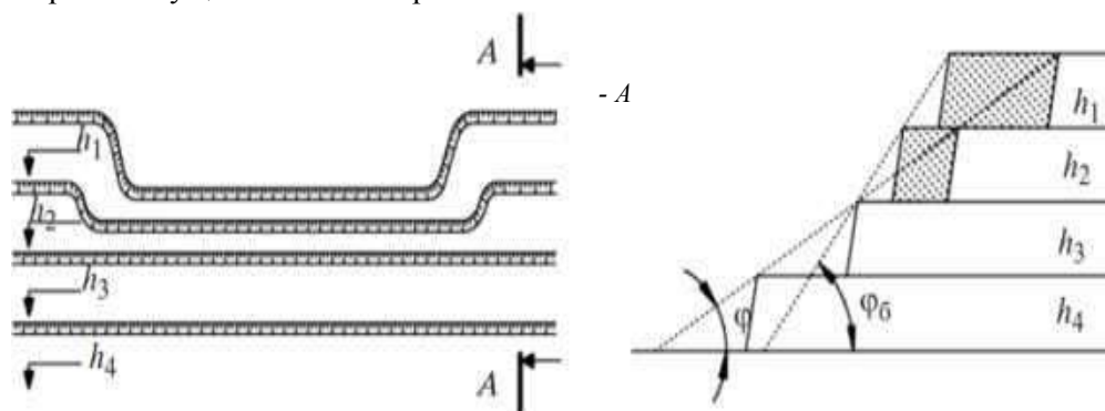
Рис. 3. Процесс формирования нерабочего борта при изменении угла наклона борта
