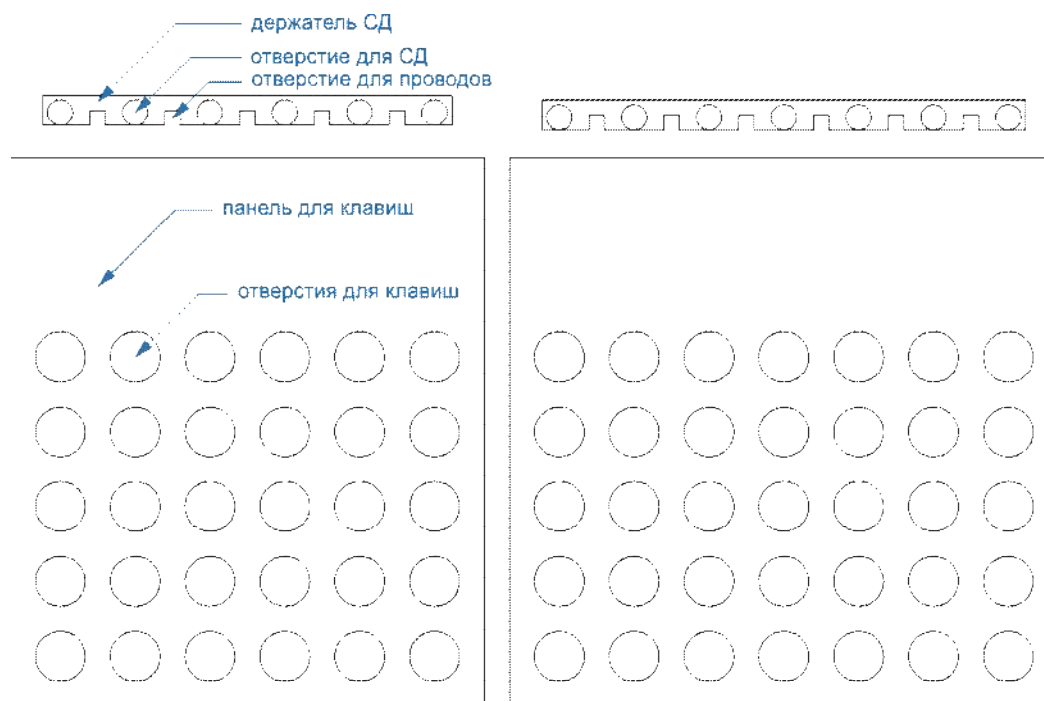
Рис. 6. Лицевая сторона верхней панели
