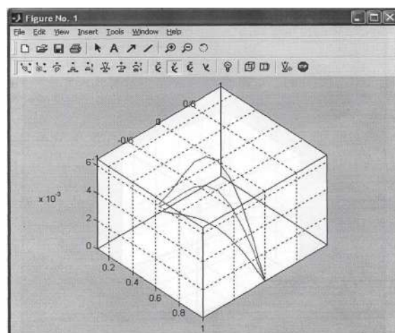
График 2. Характер движения деформации материала площади контакта в плоскости Y-Z при радиальном импульсе.
