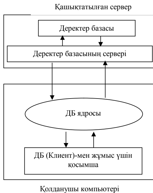
2-сурет. «Клиент-сервер» архитектурасы
