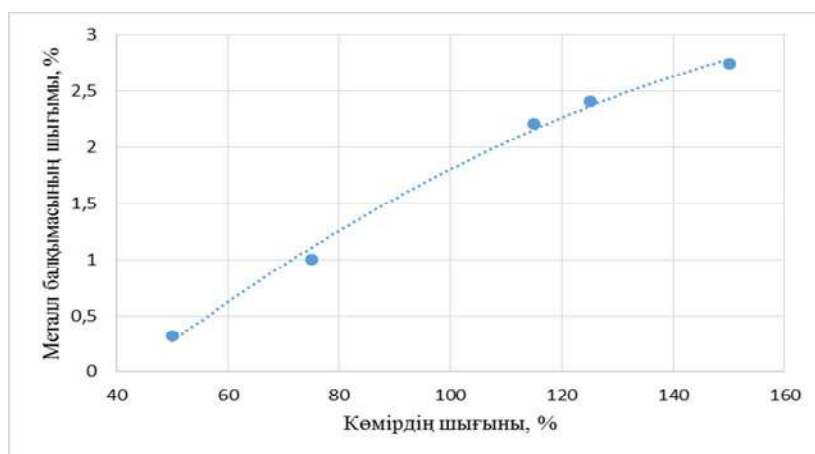
2-сурет. Тотықсыздандырғыш шығынының металл балқымасы шығымына әсері
