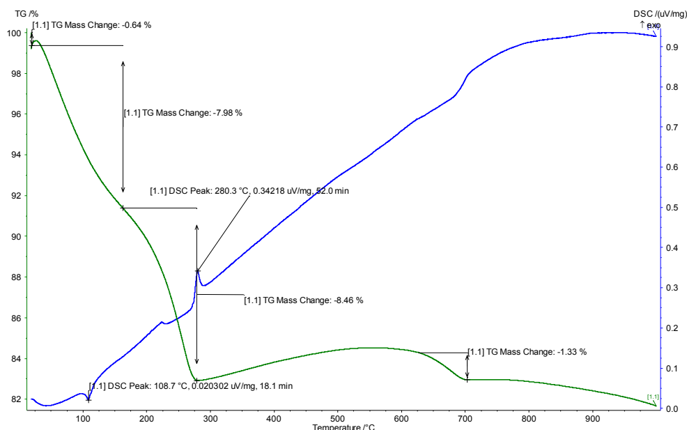
Рис. 4. Дериватограмма диспергированной смеси в течение 10 минут фосфорита Каратау и нефтяной серы
