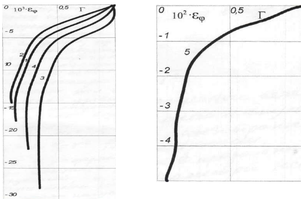
Рис.1. Распределение окружных деформации по толщине конструкции
