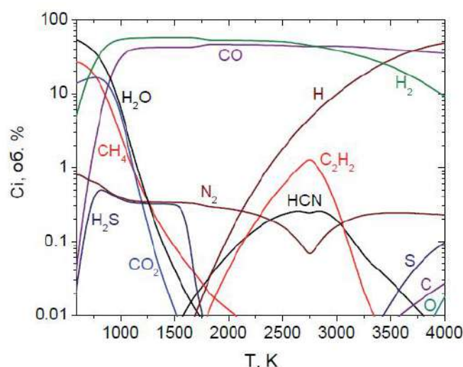
Рис. 1. Температурная зависимость концентраций органических компонентов в газовой фазе при плазменно-паровой газификации ККУ (с учетом кислорода ММУ)
