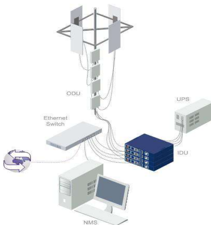
1-сурет. WiMAX базалық станциясының сұлбасы
