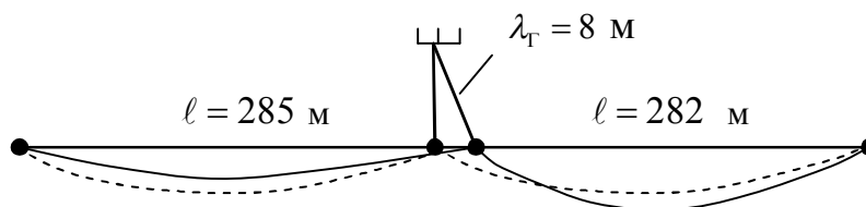
Рис. 7. 2-х пролетная система (расщепленная фаза из 3-х проводов марки АС- 300/39)
