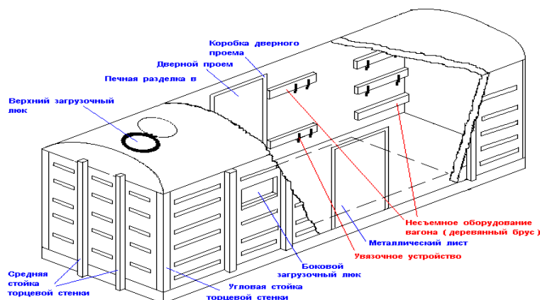
Рис. 1.1. Устройство кузова крытого вагона
