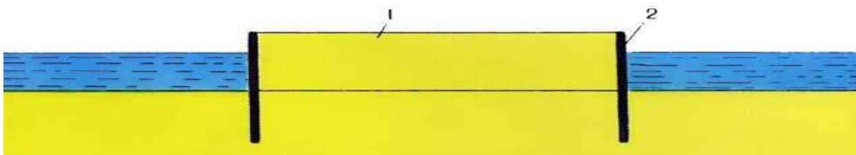
Рис. 4. Остров с металлическим (шпунтовым) ограждением: 1 - грунт; 2 - металлическое ограждение.
