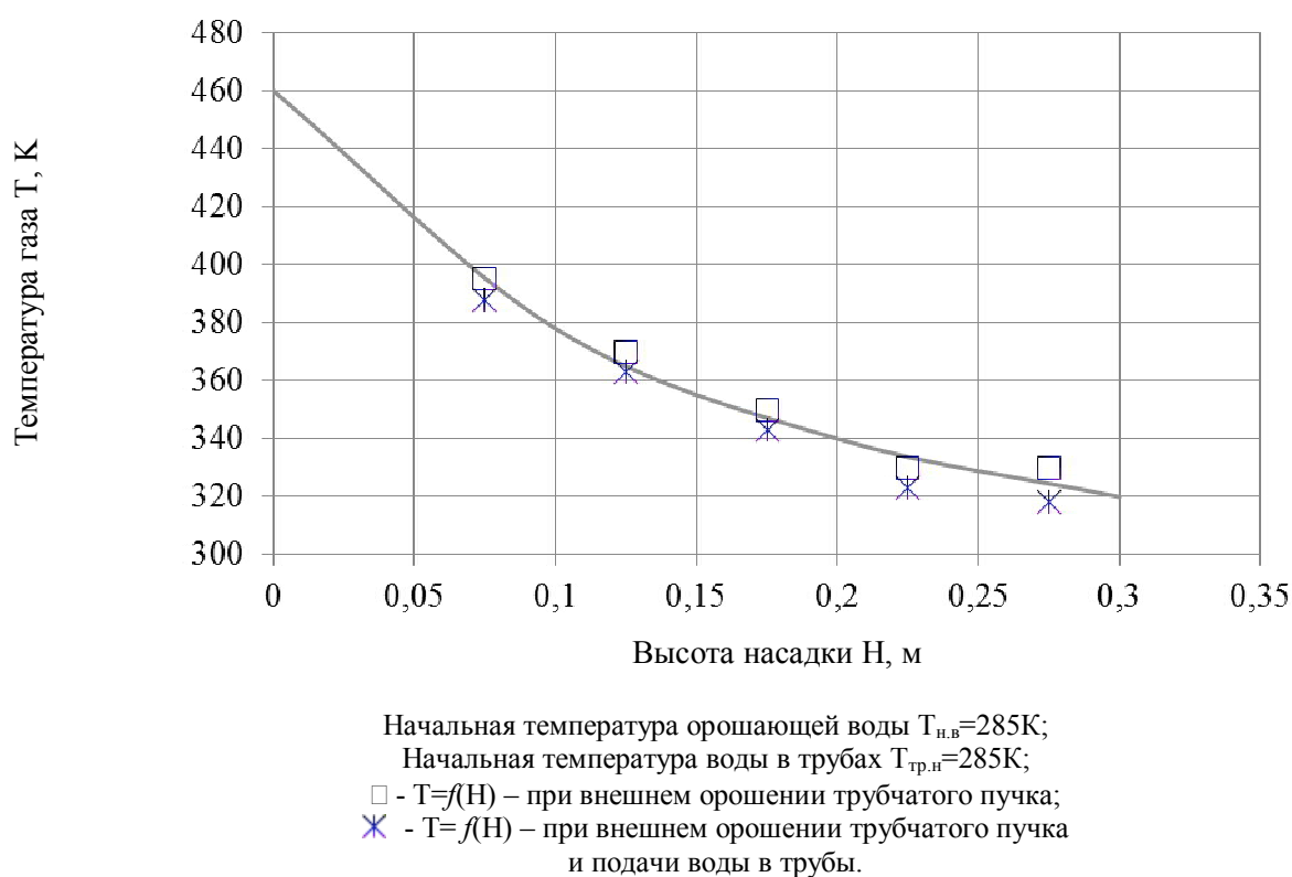
Рис. 2. Изменение температуры парогазовой смеси T по высоте аппарата H при подаче воды в трубы и внешнем орошении трубчатого пучка.
