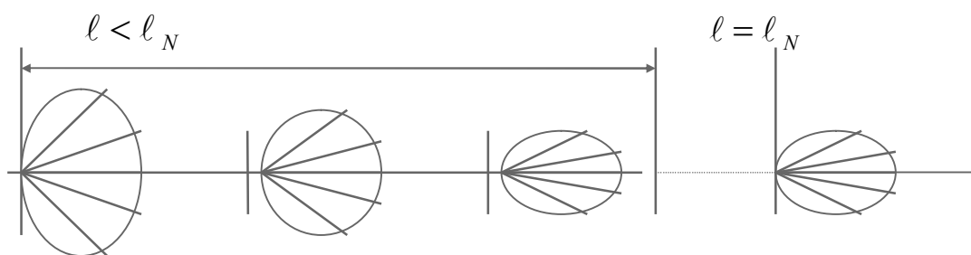
Рис.1. Деформация диаграммы излучения в световоде
