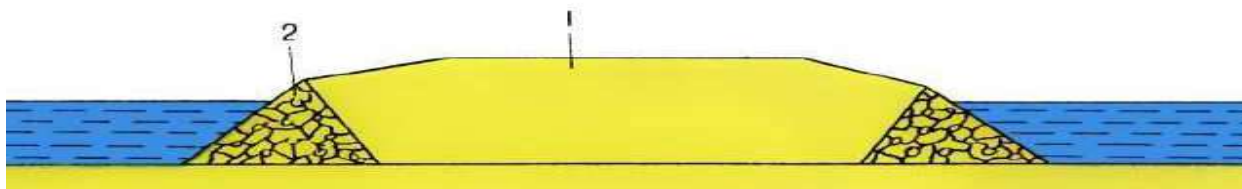
Рис. 2. Грунтовый остров с каменно-набросным ограждением: 1 -засыпка (намыв) грунта; 2 - каменнаяпризма по периметру.
