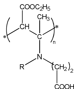
Рис. 1. Структура полимерного ПАВ CROHDA-MAA
