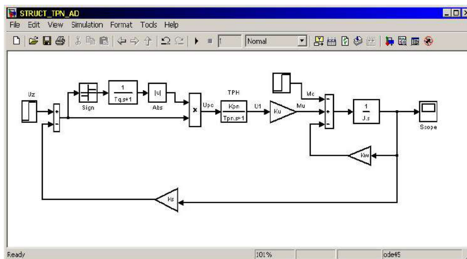
Рис. 1. Структурная схема системы ТПН – АД с обратной связью по скорости
