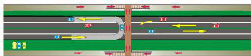
Рис. 6. Пример линейной развязки в стесненных условиях
