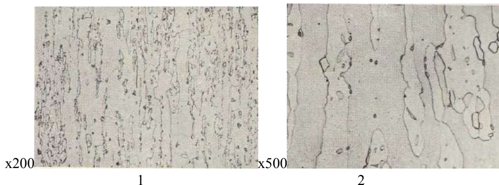
6-сурет. Хром – ванадий БА-6 болаттарының микроқұрылымы
