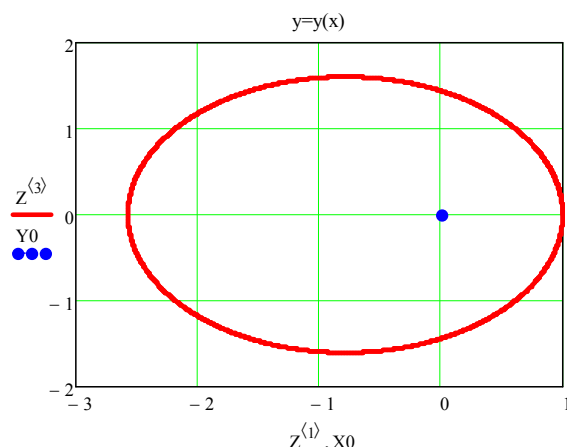
7-сурет. Центрілік күш өрісіндегі қозғалаған дененің траекториясы
