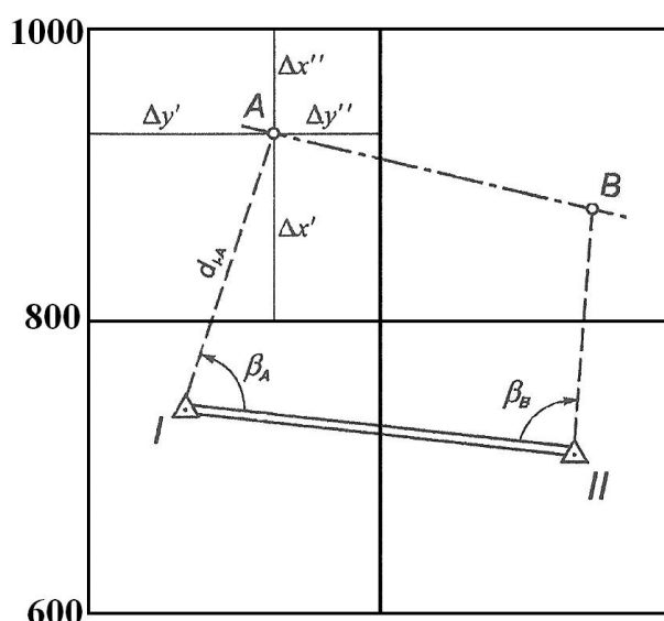
1-сурет. Бастапқы мәліметтерді дайындаудың граф-аналитикалық тәсілі
