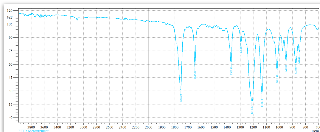
Рис. 3. ИК-спектр винилацетата
