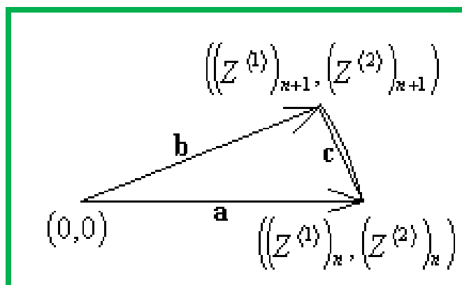
8-сурет. \Delta t уақыт аралығындағы радиус-вектордың сызатын ауданы
