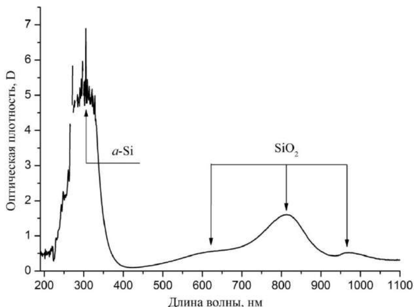
Рис. 3. Спектр поглощения (оптическая плотность) раствора синего кремнемолибденового комплекса, приготовленного из диатомита с площади «Жалпак». Максимальная оптическая плотность - 7
