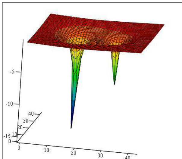
2-сурет. Потенциалдың жалпы түрі
