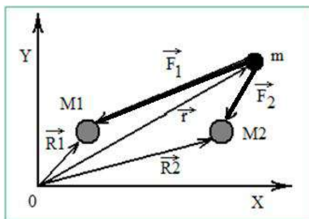
1-сурет. Үш дене туралы шектелген есептегі m дененің орны және оған M_1 және M_2 тарапынан әсер ететін күштер
