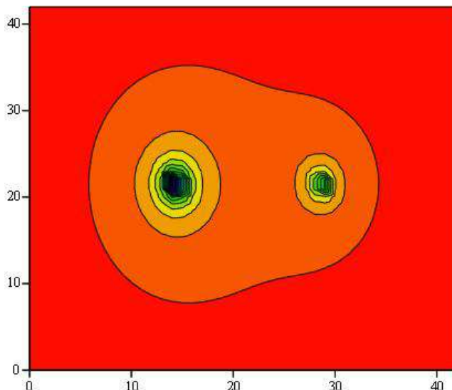
3-сурет. Потенциал сызықтарының деңгейлерінің картасы
