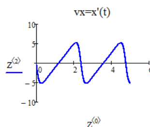
4-сурет. v_x = v(t) тәуелділігінің графигі
