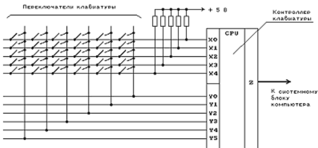
Рис. 5. Упрощенная схема клавиатуры
