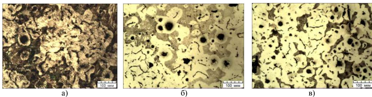
Рис. 3. Микроструктуры исследуемых образцов, x200: а) исходный образец А; б) образец Б модифицированный FC75; в) образец В модифицированный FC75+ФЧ
