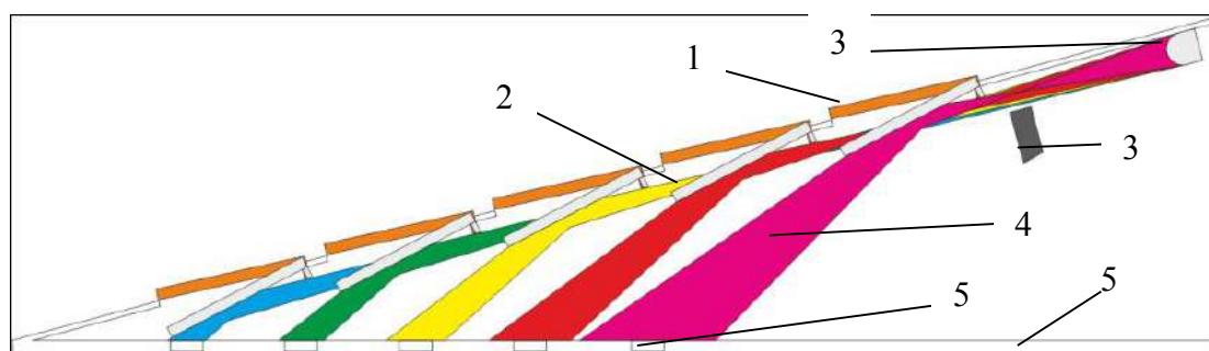
Рис. 5. Распределение света при нажатии на клавишу
