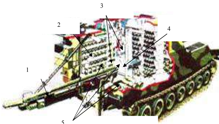
Рис. 1. Транспортно-заряжающая машина FAASV (M109ADS): 1 – транспортер, 2 – взрыватели, 3 – механизм подачи, 4 – лотки для снарядов, 5 – размещение контейнеров.
