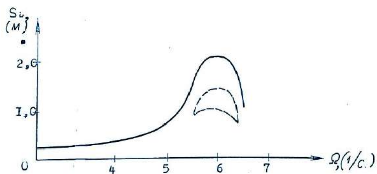
Рис. 5. Амплитудно-частотная характеристика колебаний нити на частоте суммарного тона при \gamma=3
