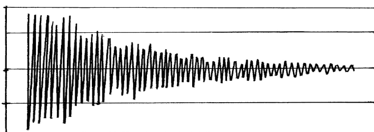
3-сурет Хром-молибден болатының БА - 4 соққыш-шардың екпіні әсерінен дыбыс импульсінің азаю осцилограммасы көрсетілген
