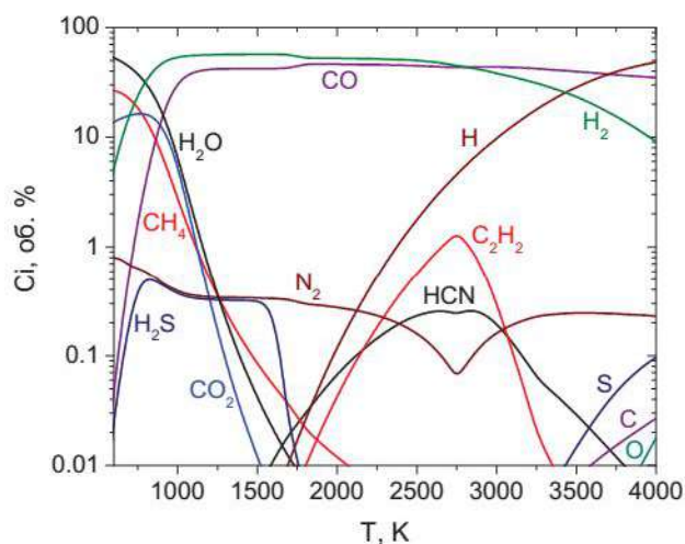
Рис. 2. Температурная зависимость концентраций органических компонентов в газовой фазе при комплексной переработке угля
