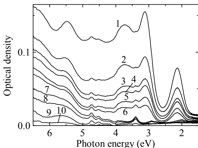
Рис. 1. Спектры индуцированного оптического поглощения облученного при комнатной температуре рентгеновскими лучами кристалла \text{CaF}_2 , измеренные непосредственно после облучения (1) и после промежуточных нагревов до температур: 380 К (2), 410 К (3), 450 К (4), 490 К (5), 520 К (6), 570 К (7), 660 К (8), 823 К (9), 1023 К (10). Измерения оптического поглощения проводились при комнатной температуре.
