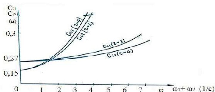
Рис. 1. Зависимость амплитуд гармонических составляющих C_{i1} и C_{i2} от суммарной частоты \Omega = \omega_1 + \omega_2
