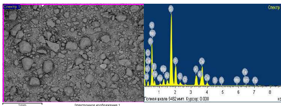
Рис. 1. Минералогический состав и микроструктура фосфорного шлама
