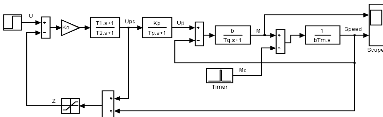
Рис. 1. Структурная схема замкнутой системы ПЧ – АД
