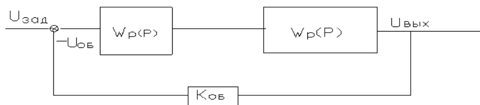
Рис. 4. Структурная схема системы стабилизации
