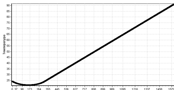
1.2-сурет. Сырық ұзындығы бойынша температураның таралу заңдылығы
