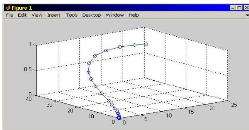
Рис. 3. Фазовая траектория динамики замкнутой системы ТПН-АД
