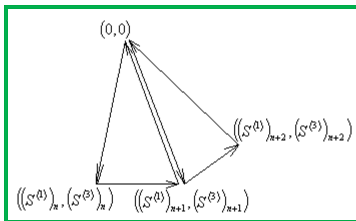
9-сурет. Гравитациялық центрлік күш өрісінде қозғалған дененің траекториясын салуға қажетті алгоритм
