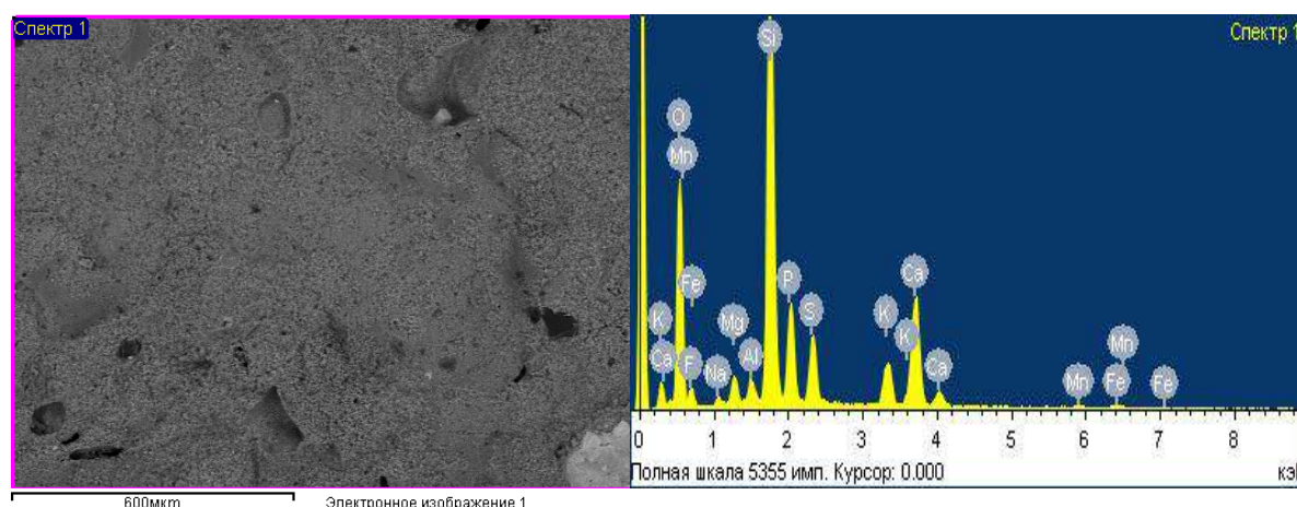
Рис. 2. Минералогический состав и микроструктура комплексного полимерсодержащего органоминерального удобрения суперфосфата с КАС
