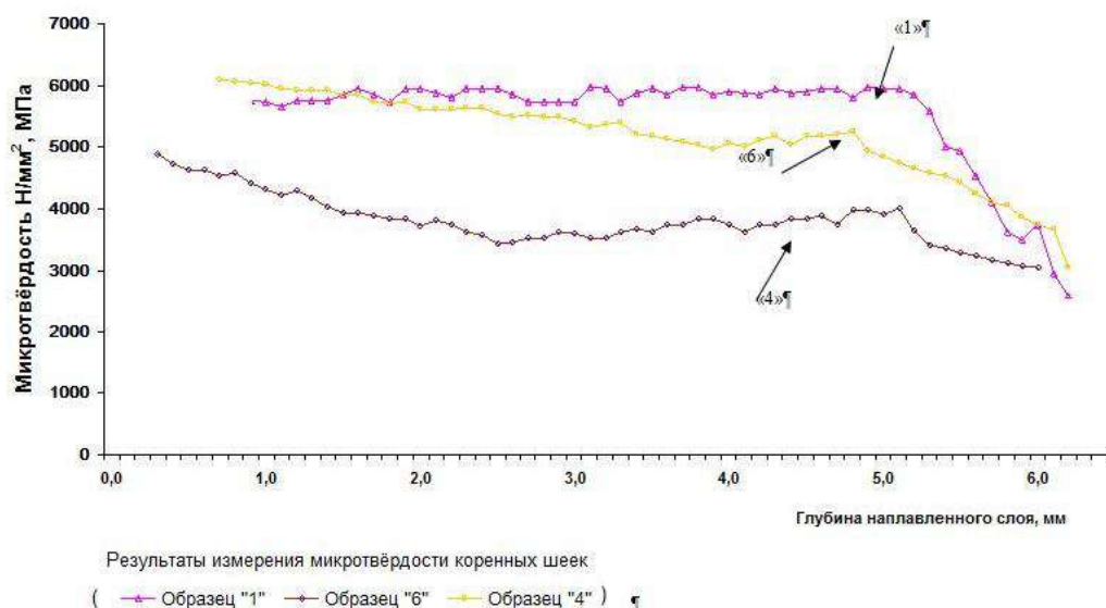
Рисунок 4 – Графики зависимости микротвёрдости коренных шеек коленчатых валов от глубины наплавленного слоя
