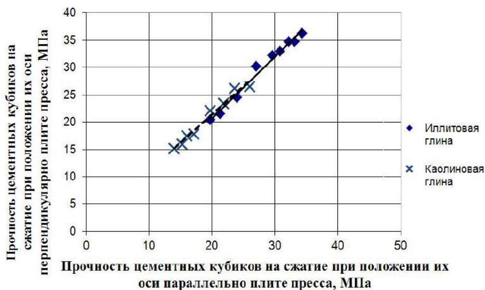
Рис. 5. Прочность образцов тампонажного камня, содержащих активные примеси, при испытаниях на одноосное сжатие и различном их пространственном положении
