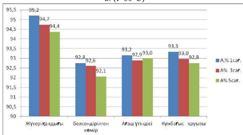
1-сурет. Адсорбенттердің уақытқа байланысты тазарту дәрежелері, %
