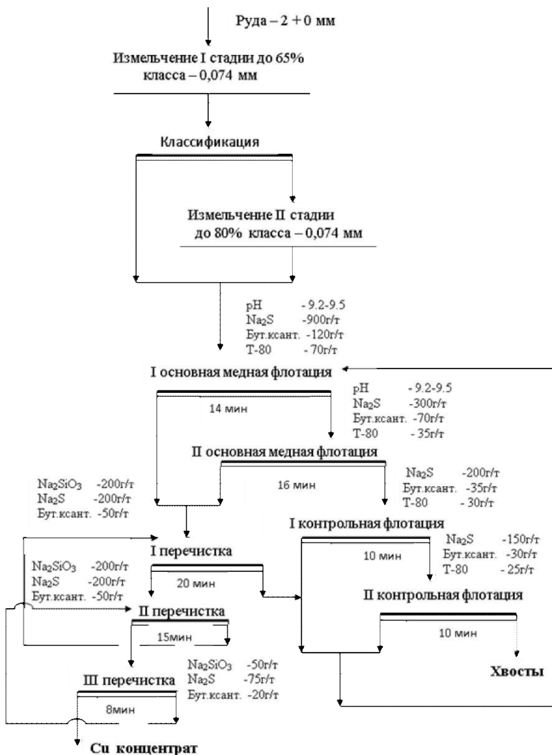
Рис. 3. Рекомендуемая схема флотации
