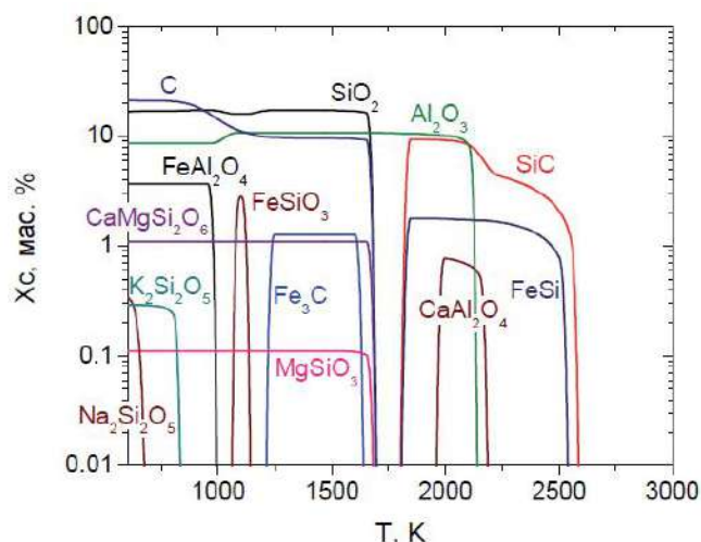
Рис. 3. Температурная зависимость концентраций компонентов конденсированной фазы при плазменно-паровой газификации ККУ (с учетом кислорода ММУ)
