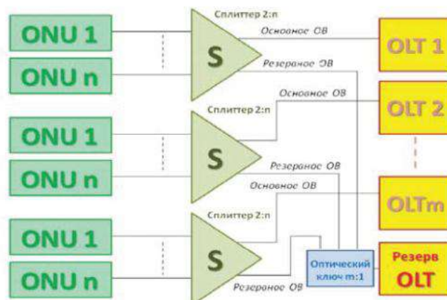
Рис. 2.5. Схема резервирования. Тип В с использованием оптического ключа типа m:1
