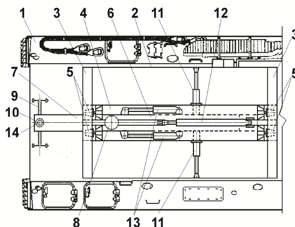
Рис. 5. Транспортно-заряжающая машина на базе МТ-ЛБу (вид сверху): 1 – базовая машина на гусеничном шасси, 2 – корпус боевой укладки, 3 – направляющие, 4 – каретка, 5 – ролики, 6 – выдвижная стрела, 7 – поворотная секция, 8 – шарнир, 9 – устройство для захвата контейнера с боевым комплектом, 10 – шарнир, 11 – гидроцилиндры поперечного перемещения каретки, 12 – гидроцилиндр «выдвижения-втягивания» стрелы, 13 – гидроцилиндры управления поворотной секцией, 14 – гидроцилиндр «подъема- опускания».
