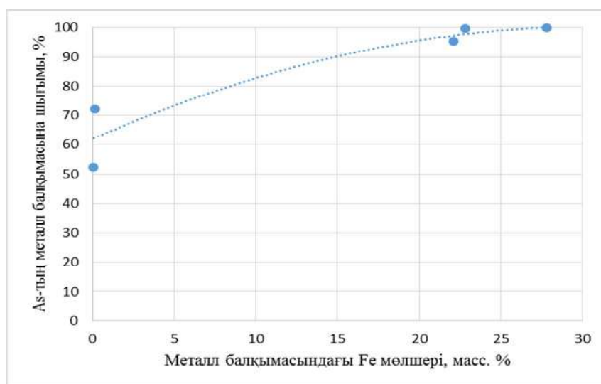
5-сурет. Мышьяқтың қорытпаға бөлініп алынуының қорытпадағы темір мөлшерінен тәуелділігі
