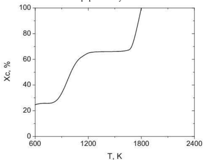
Рис. 5. Температурная зависимость степени газификации угля при его комплексной переработке
