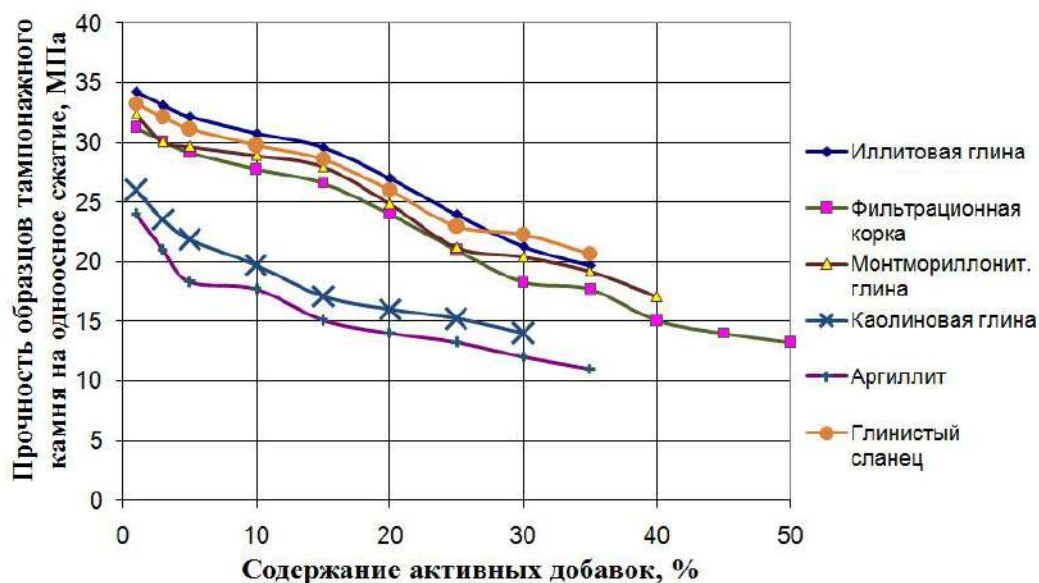
Рис. 4. Прочность образцов тампонажного камня, содержащих активные примеси, при испытаниях на одноосное сжатие
