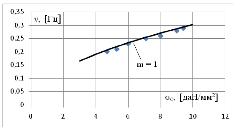
Рис. 8. Зависимость частоты колебаний 2-х пролетной системы от начального напряжения.
