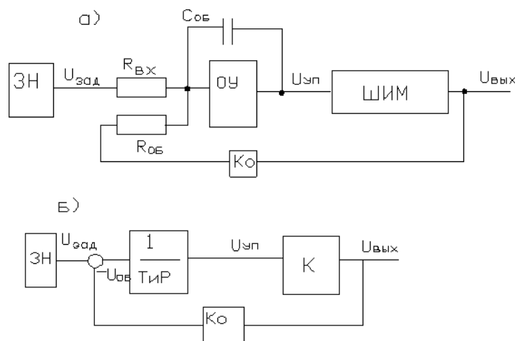
Рис. 6. Схема силовой части импульсного регулятора постоянного напряжения (а) и структурная схема системы стабилизации (б).
