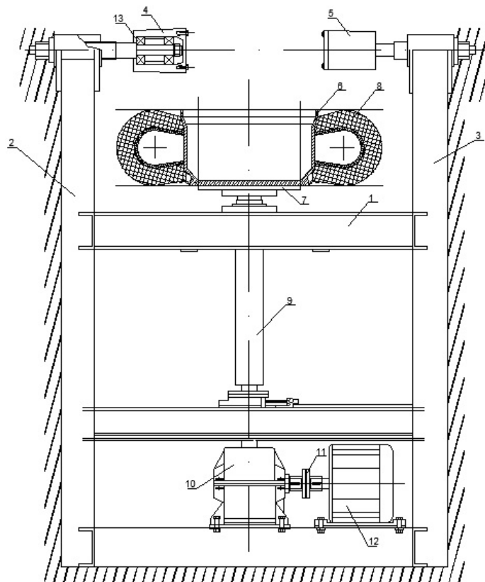
Рис. 1. Стенд для демонтажа пневмошин
