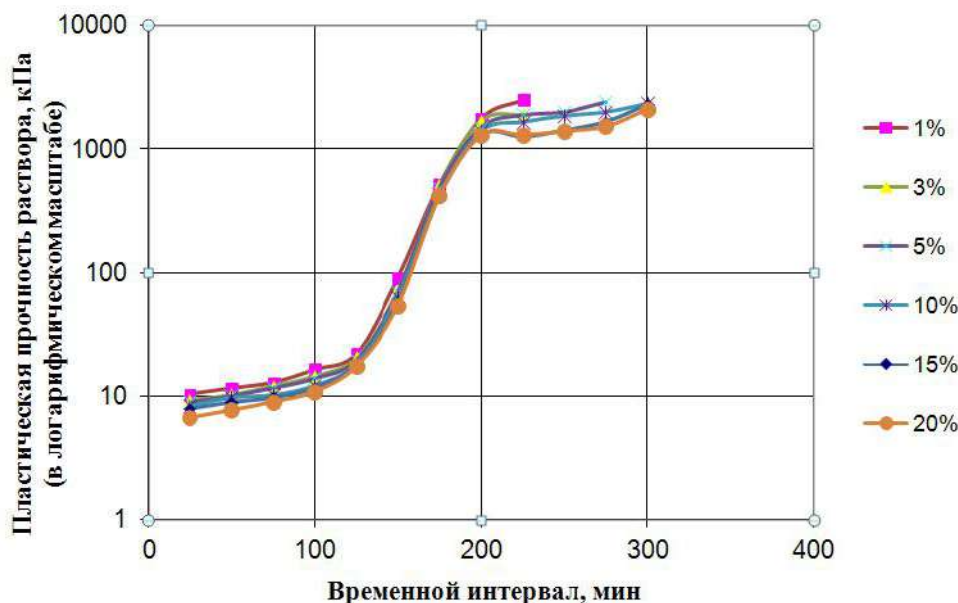
Рис. 3. Изменение пластической прочности тампонажного раствора при введении в него монтмориллонитовой глины
