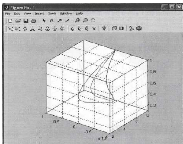
График 1. Характер движения деформации материала площади контакта в плоскости Y-Z при линейном импульсе.
