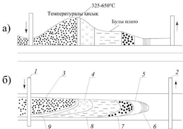
а – қабаттағы температуралық аймақтар; б – процестің таралу аймақтары; 1,2 – айдау және алу ұңғымалары; 3,4,7,8 – сәйкесінше жанған, буланған, конденсация және бу аймақтары; 5 – жеңіл көмірсутектер; 6 – мұнай білігі; 9 – жану фронты.
