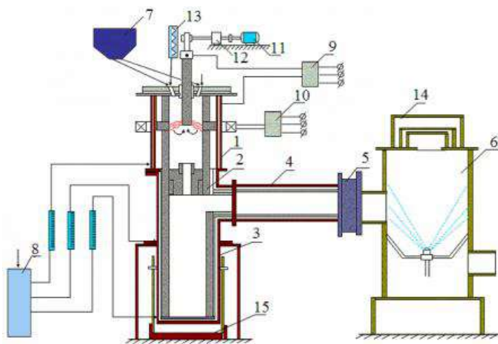
Рис. 1. Схема плазменной установки для газификации углей.
