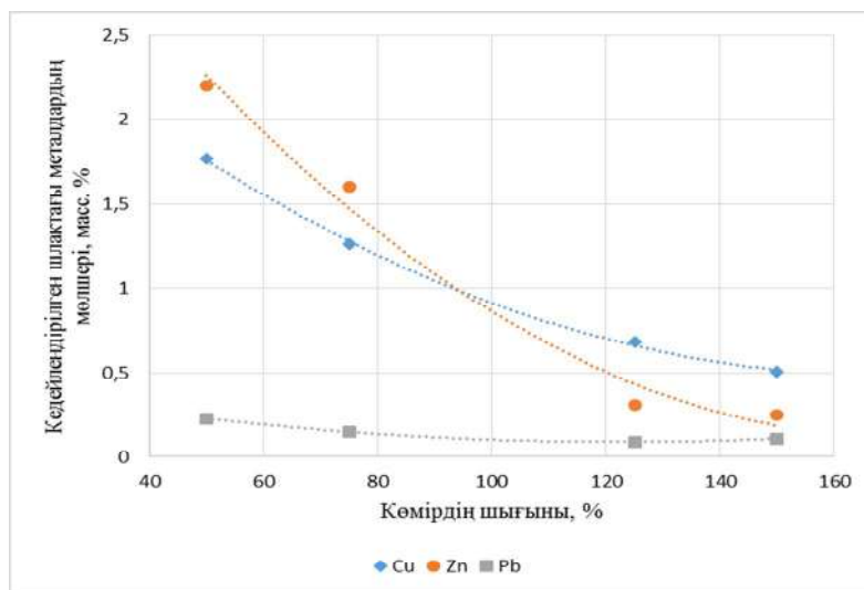
4-сурет. Шлактағы түсті металдардың мөлшерінің көмірдің шығынынан тәуелділігі
