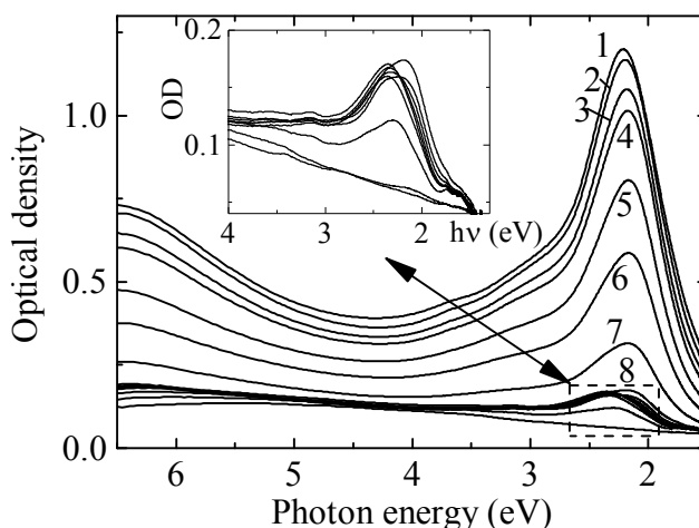
Рис. 2. Спектры индуцированного оптического поглощения облученного при комнатной температуре ионами \text{He}^{132} с флюенсом 1 \times 10^{14} ион/см 2 кристалла \text{CaF}_2 , измеренные непосредственно после облучения (1) и после промежуточных нагревов до температур: 410 К (2), 440 К (3), 470 К (4), 500 К (5), 520 К (6), 540 К (7), 560–773 К (8). Измерения оптического поглощения проводились при комнатной температуре.
