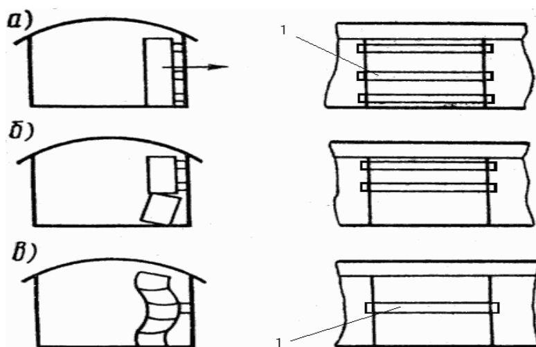
Рис. 1.4. Установка досок ограждения дверного проема от навала груза 1 - доска ограждения
