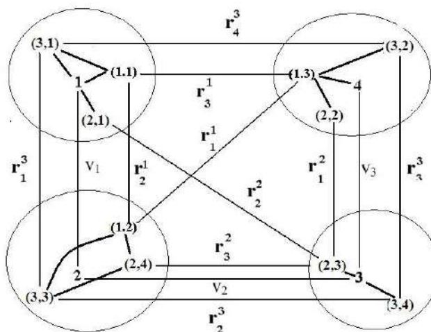
Рис. 2. Сумма графов всех сетей S-гиперсети HS
