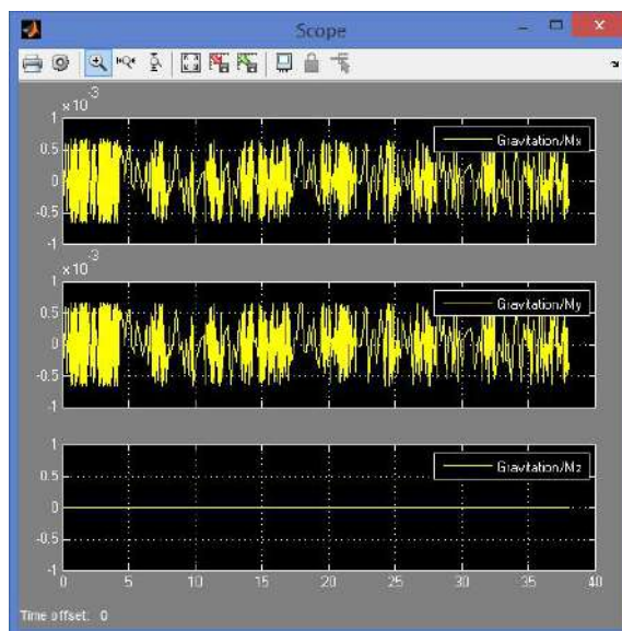
Рис. 7. Графики значений гравитационных моментов
