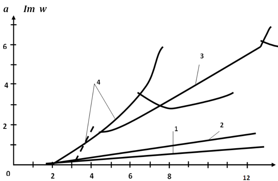
Рис.1,б. Зависимость \text{Im } \omega от волнового числа k
