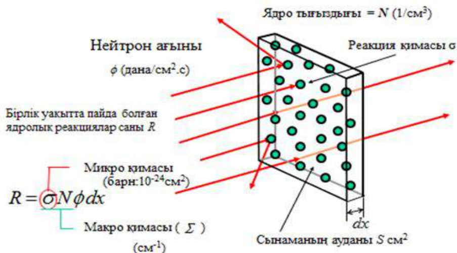
1-сурет. Нейтрондардың нысана ядроларымен реакциялану қимасының сұлбасы
