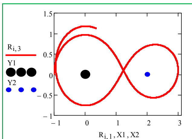
4-сурет. Дененің қозғалыс траекториясы
