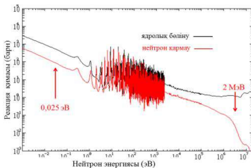
2-сурет. Нейтрон энергиясының U^{235} реакция қимасына әсері
