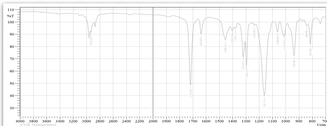
Рис. 2. ИК-спектр бутилметакрилата
