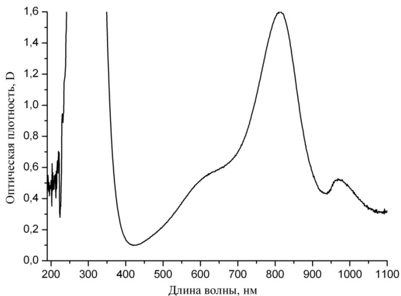
Рис. 4. Спектр поглощения (оптическая плотность) раствора синего кремнемолибденового комплекса, приготовленного из диатомита с площади «Жалпак». Максимальная оптическая плотность – 1,7
