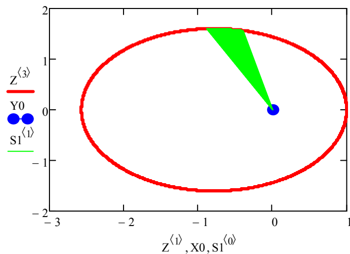
10-сурет. Центрілік күш өрісіндегі қозғалаған дененің траекториясын сол дененің радиус-векторы сызған ауданмен бірге салу
