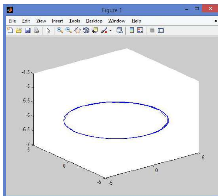
Рис. 4. Трехмерная модель движения КА под влиянием гравитационных моментов
