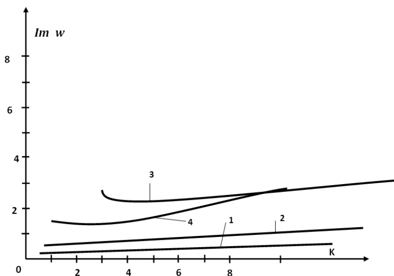
Рис. 2,б. Зависимость \text{Im } \omega от волнового числа k
