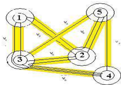
Рис. 3. Планарная гиперсеть
