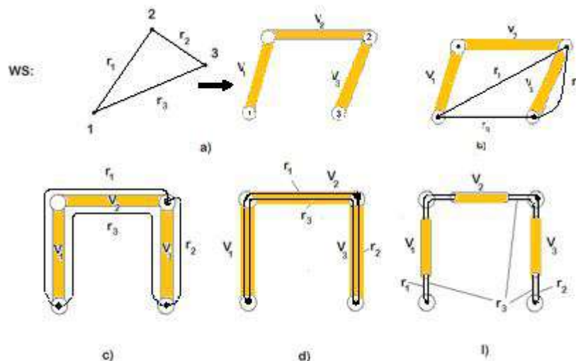
Рис. 7. Примеры топологических взаимосвязей ребер и вершин различных сетей S-гиперсети H = (WS, PS)
