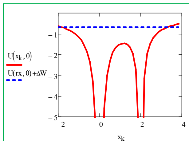
5-сурет. OXy жазықтығындағы U(x,y) потенциалының қимасы.
