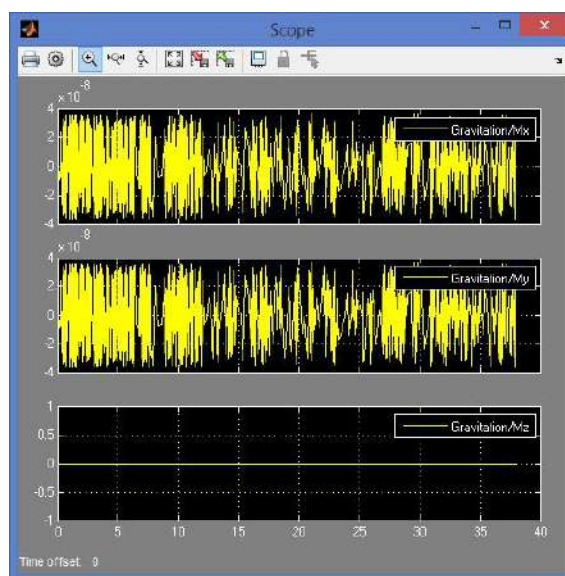
Рис. 6. Графики значений гравитационных моментов
