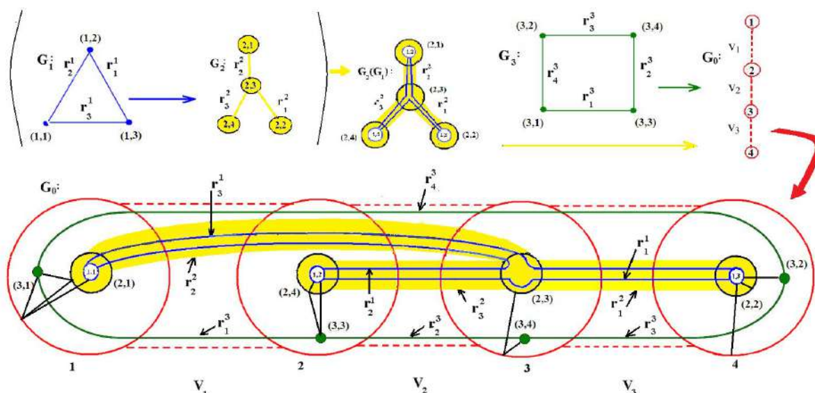
Рис. 1. Пример гиперсети
