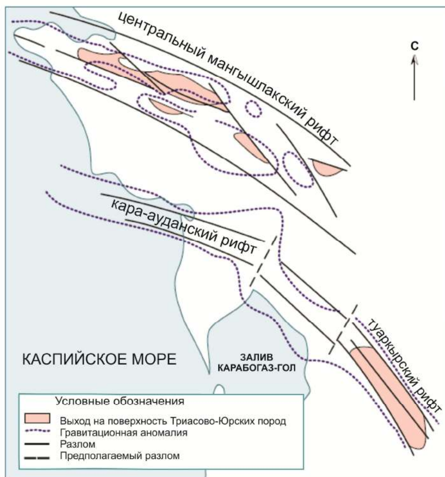
Рис. 2. Тектоническая схема Триасовых рифтовых систем (по Мурзагалиеву 1996 г.)
