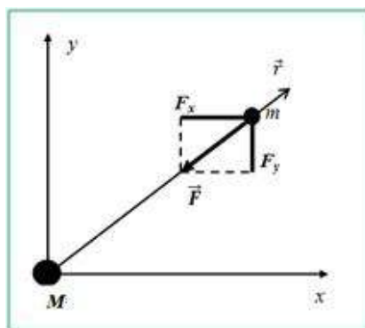
1-сурет. Центрілік күш өрісінде орналасқан дене
