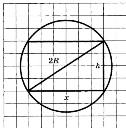
Рис. 1. Прямоугольник, вписанный в окружность радиусом R .
