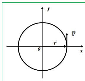
2-сурет. Центрілік күш өрісіндегі дененің жылдамдығы
