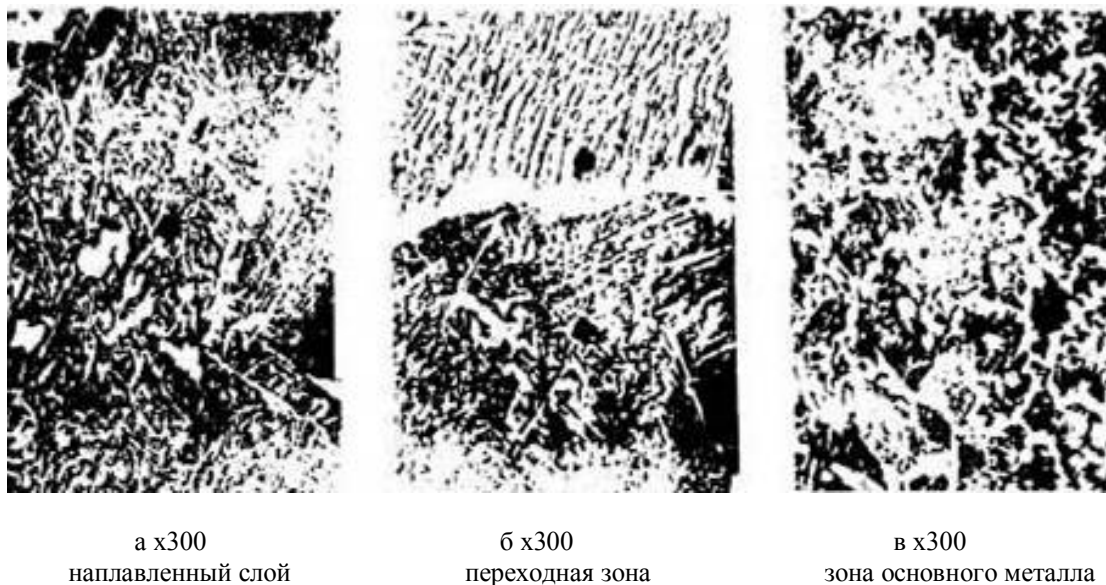
Рис. 3. Микроструктура наплавленного металла (образец «б», шатунная шейка, 15 ГСТЮЦА + СОРМАИТ)
