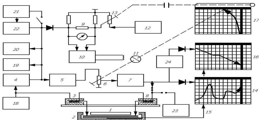
1-сурет. Ішкі үйкеліс пен тығыздық модулін үздіксіз бекіткіш автоматты құрылғысының блок-схемасы 1 – қыздырғыш (суытқыш) құрылғы; 2 – үлгі; 3 – тербеліс датчигі; 4 – күшейткіш; 5 – фильтр; 6 – потенциометр; 7 – қуатты үдеткіш; 8 – тербелісті қоздырғыш; 9 – салыстыру блогы; 10 – сервокүшейткіш (КСП-4); 11 – сервоқозғалтқыш; 12 – кернеулерді тұрақтандырғыш блогы; 13 – потенциометр; 14 – өздігіненжазғыш; 15 – термобу; 16 – өздігіненжазғыш; 17 – потенциометр; 18 – лампалық вольтметр; 19 – осциллограф; 20 – жиілік өлшеуіш; 21 – дискриминатор; 22 – импульс есептеуіш; 23 – генератор; 24 – блок.
