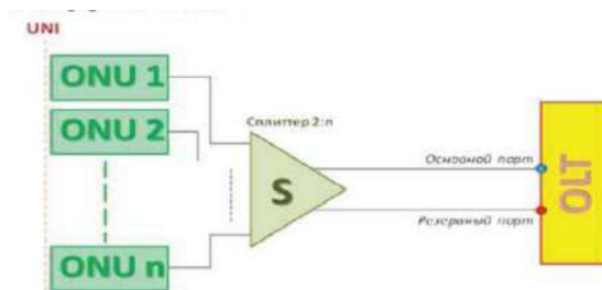
Рис. 2.2. Схема резервирования. Тип В
