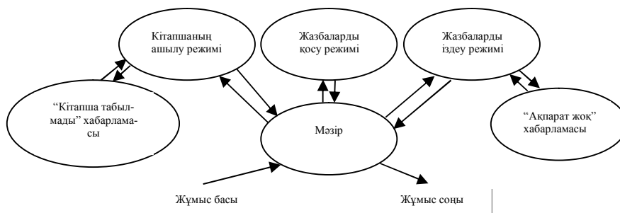
6-сурет. Қолданушы интерфейсі жағдайының толық диаграммасы.
