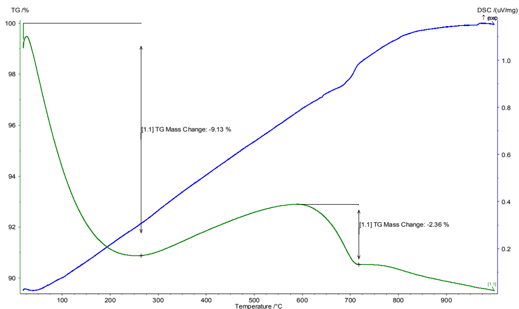
Рис. 2. Дериватограмма фосфорита Каратау
