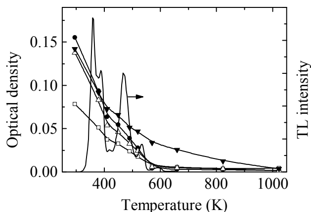
Рис. 3. Зависимость радиационно-индуцированного оптического поглощения от температуры промежуточных нагревов для соответствующих спектральных областей: 2.13 эВ ( \square ), 3.12 эВ ( \bullet ), 3.73 эВ ( \Delta ) и 5.5 эВ ( \blacktriangledown ) и кривая ТСЛ (правая шкала) для X-облученного при комнатной температуре кристалла \text{CaF}_2 . Оптическое поглощение измерено при комнатной температуре.
