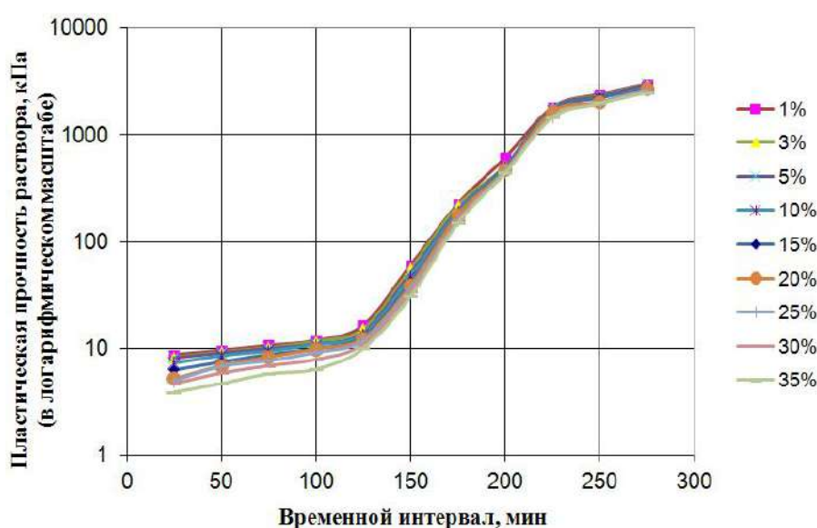
Рис. 2. Изменение пластической прочности тампонажного раствора при введении в него глинистого сланца
