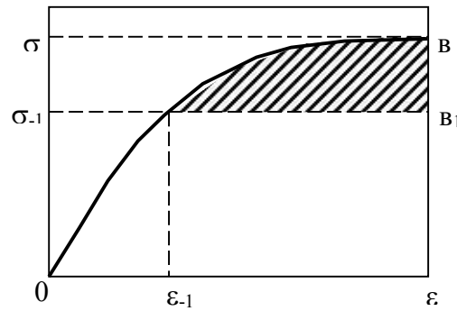
Рис. 1. Снижение прочности динамической нагрузки
